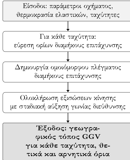
Σχήμα 23: Διαδικασία δημιουργίας διαγράμματος GGV.
