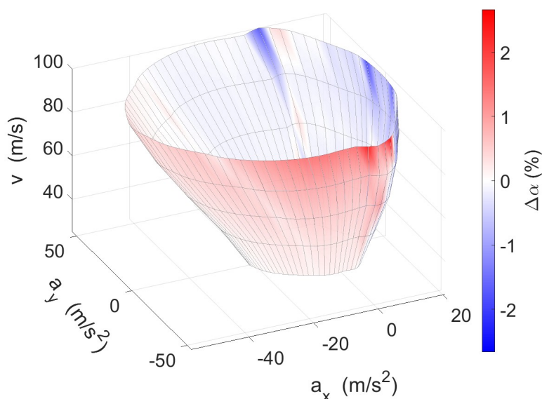
Σχήμα 26: Ποσοστιαίο σφάλμα προσέγγισης κοινής θερμοκρασίας - στις θετικές τιμές υπερεκτιμώνται οι επιδόσεις του οχήματος.
