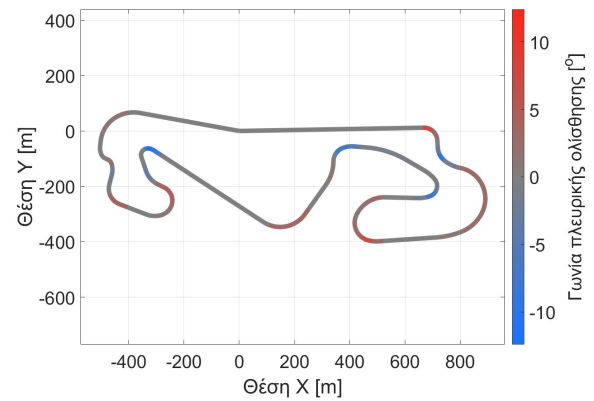
(β) Γωνία πλευρικής ολίσθησης
