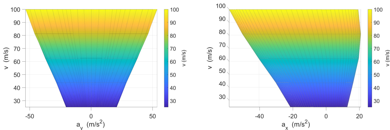
(α) Εμπρόσθια προβολή διαγράμματος επιδόσεων
