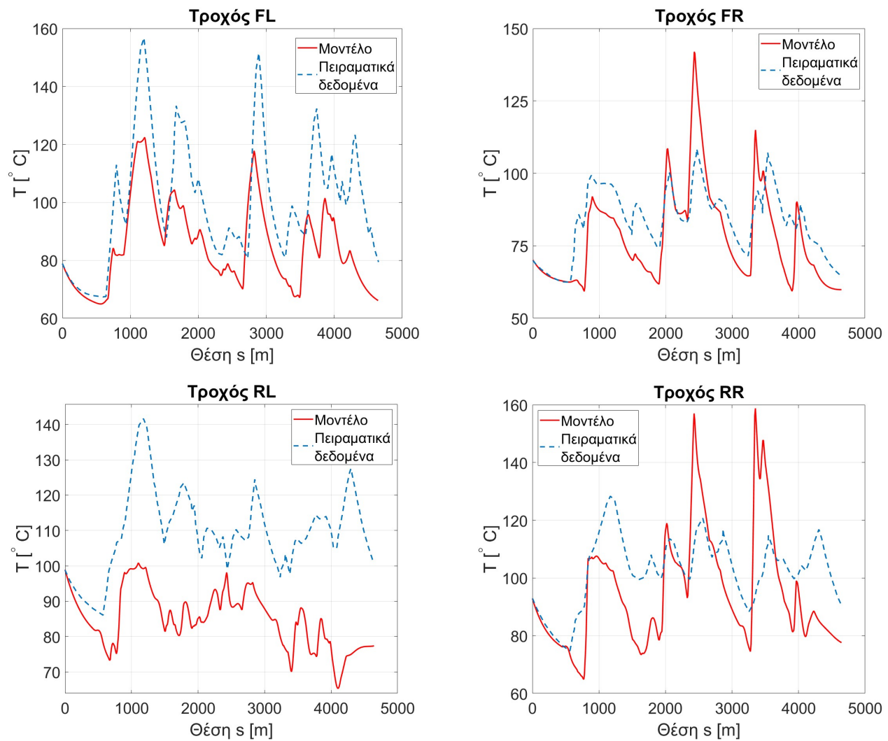
Σχήμα 30: Σύγκριση θερμοκρασίας μοντέλου με πειραματική σε γύρο της πίστας Circuit de Barcelona - Catalunya
