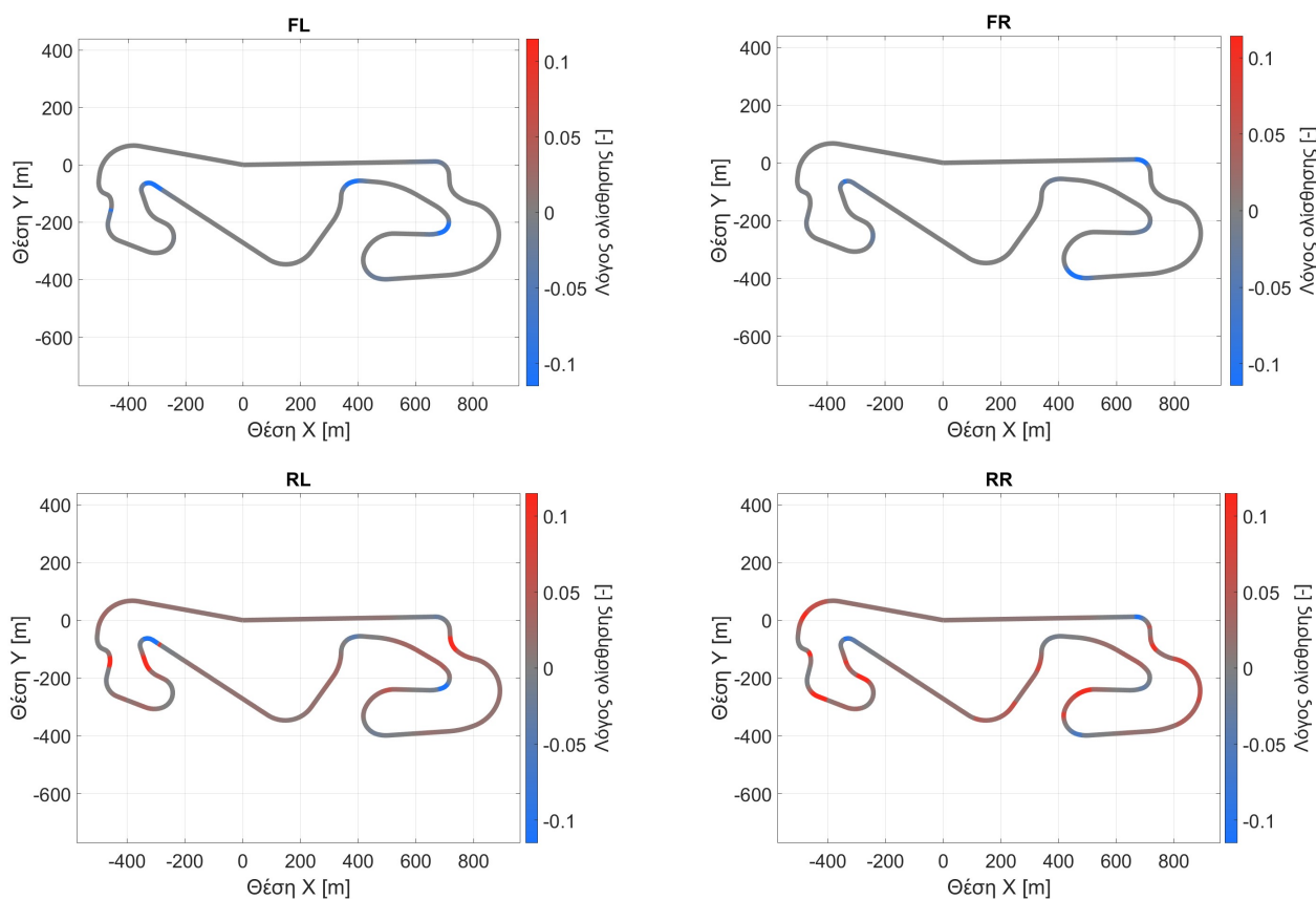
Σχήμα 20: Ενδεικτικά αποτελέσματα λόγου ολίσθησης σε γύρο της πίστας Circuit de Barcelona - Catalunya
