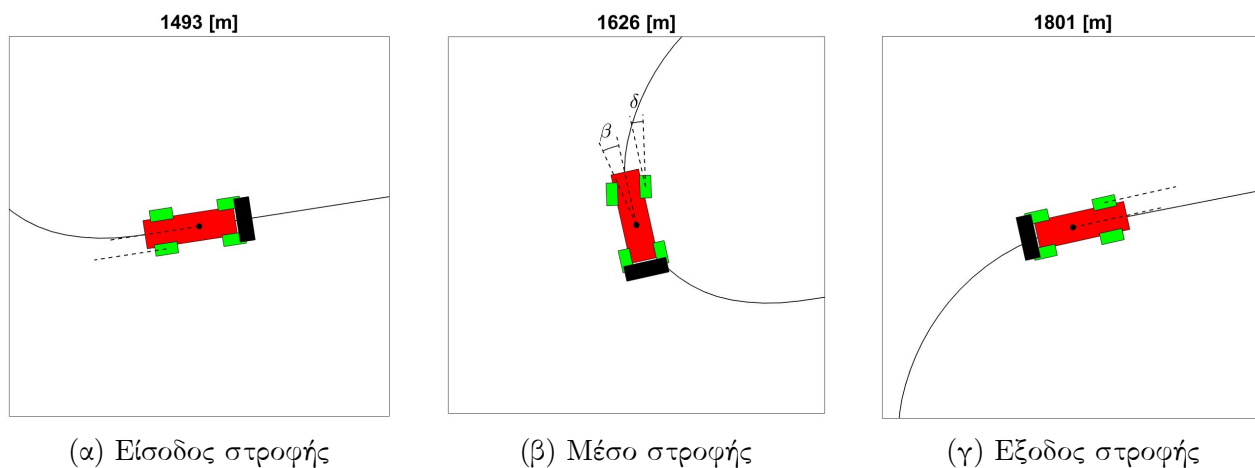
Σχήμα 19: Ενδεικτική σχηματική αναπαράσταση αποτελεσμάτων επίλυσης της κατάστασης οχήματος.
