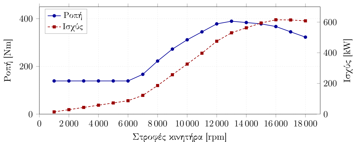
Σχήμα 29: Καμπύλη ροπής κινητήρα.
