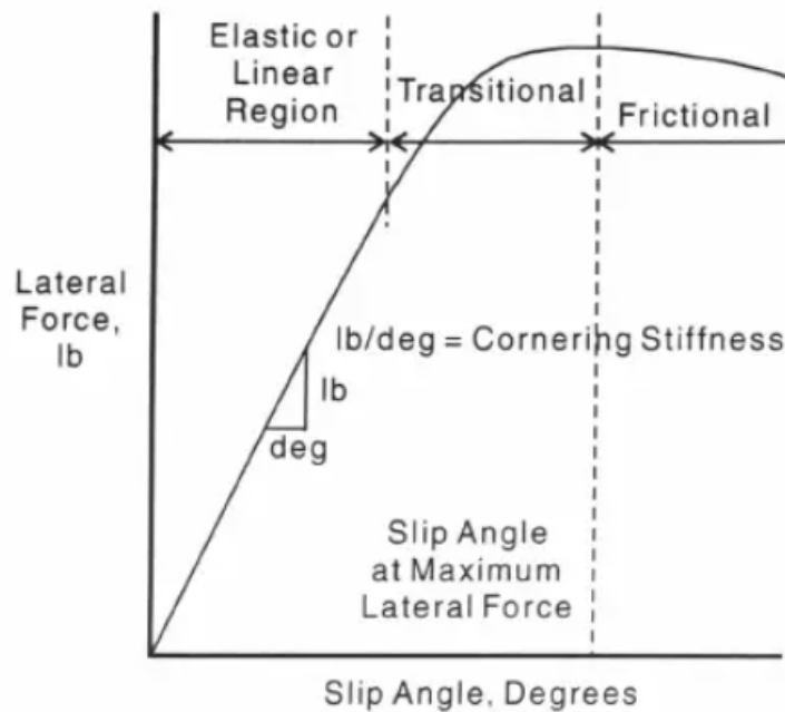
Σχήμα 2: Περιοχές προσκόλλησης - ολίσθησης [8]
