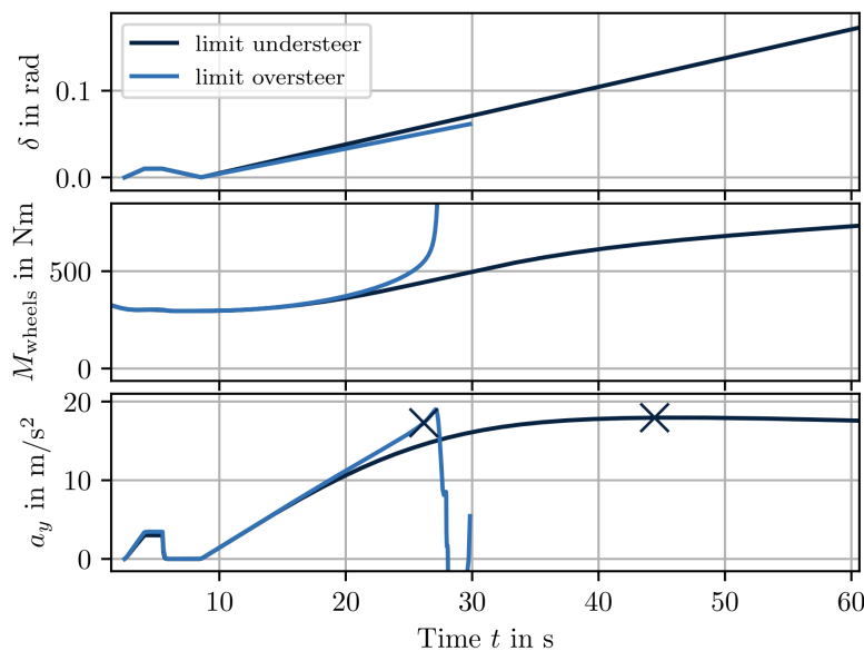
Σχήμα 25: Μέθοδος εύρεσης μέγιστης πλευρικής επιτάχυνσης [28]
