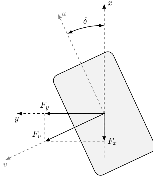
Σχήμα 17: Ανάλυση δυνάμεων κατευθυντήριου τροχού – επαγόμενη αντίσταση
