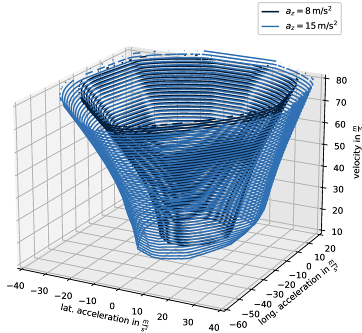
Σχήμα 22: Ενδεικτικό διάγραμμα επιδόσεων (GGV) [28]
