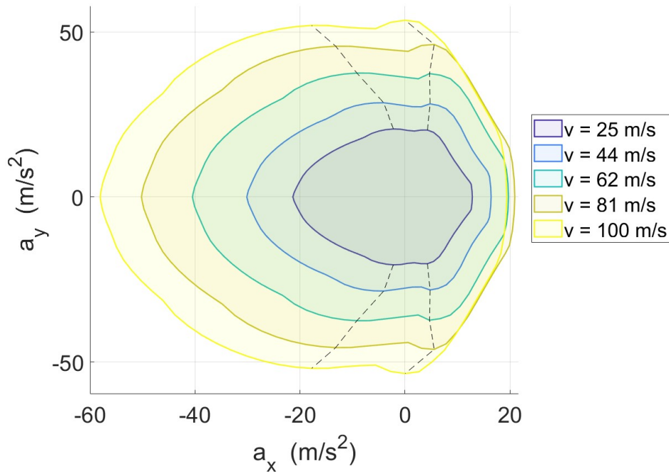
Σχήμα 28: Μορφή διαγράμματος επιδόσεων σε διαφορετικές ταχύτητες
