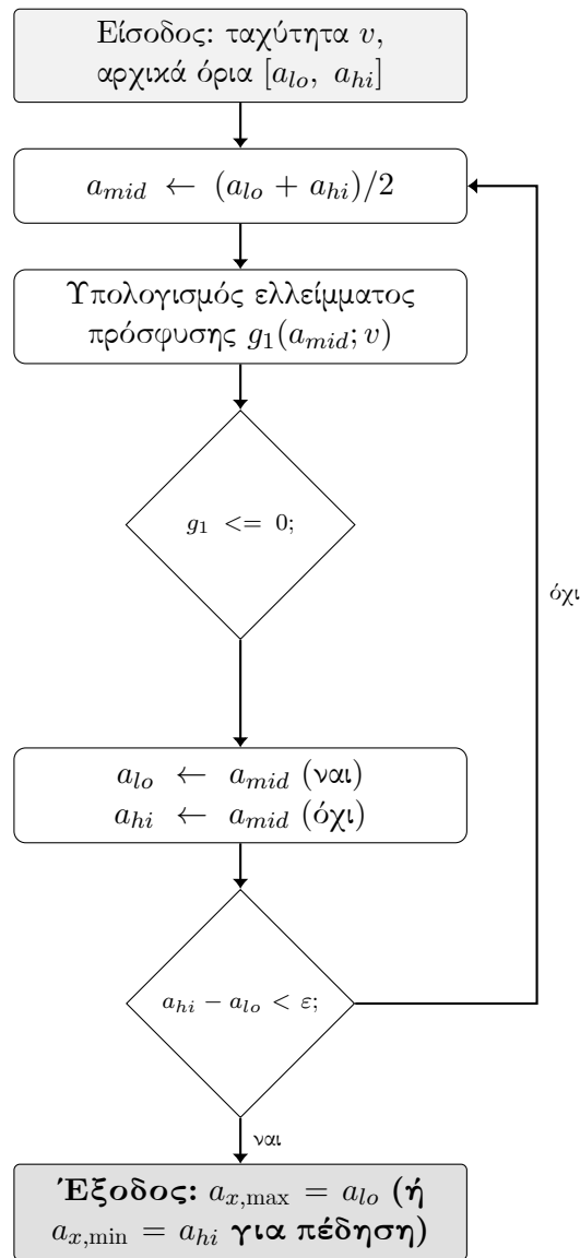
Σχήμα 24: Διάγραμμα ροής – δυαδική αναζήτηση διαμήκους ορίου πρόσφυσης σε ευθεία.
