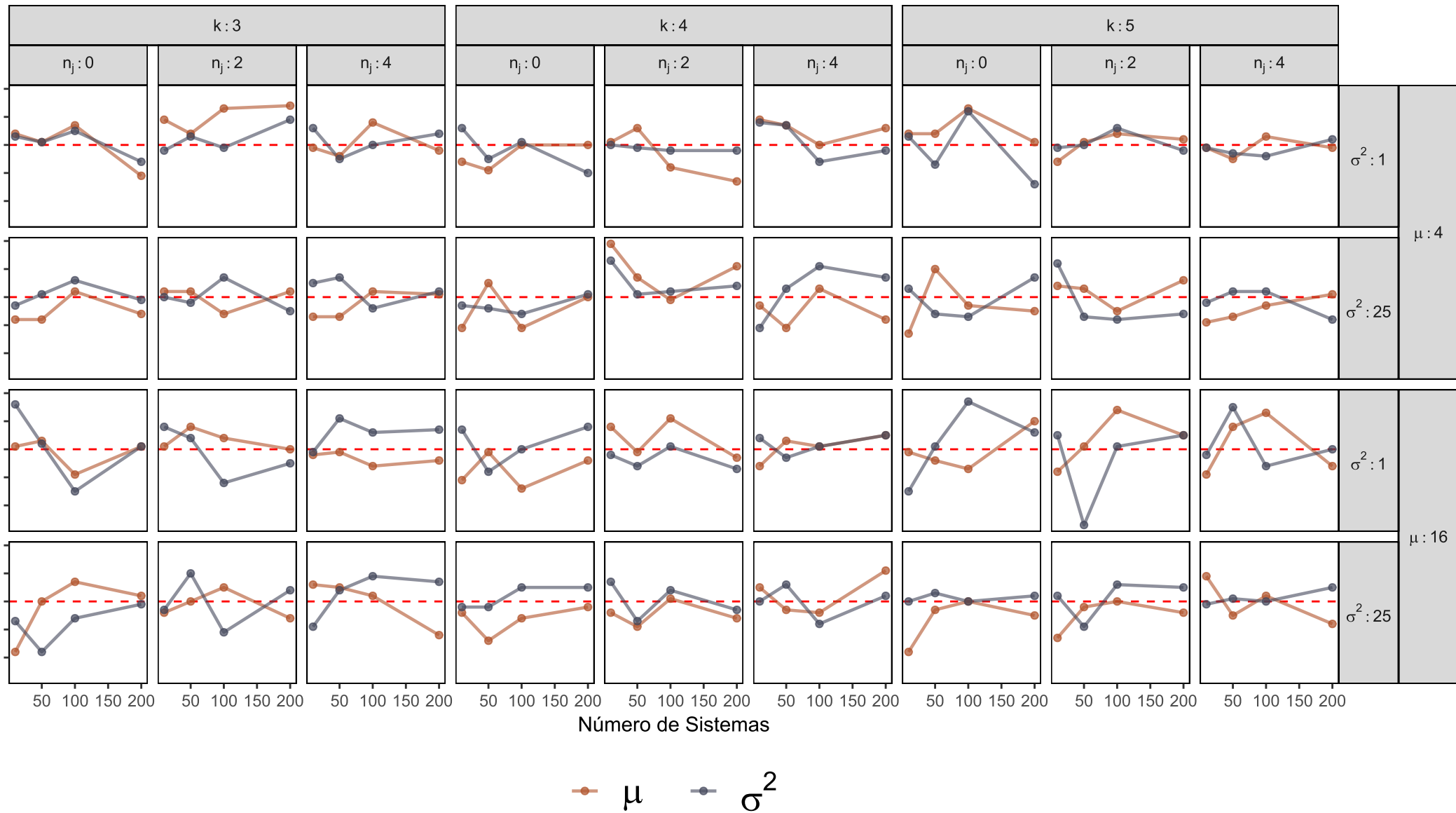
Probabilidade de Cobertura (95%)
