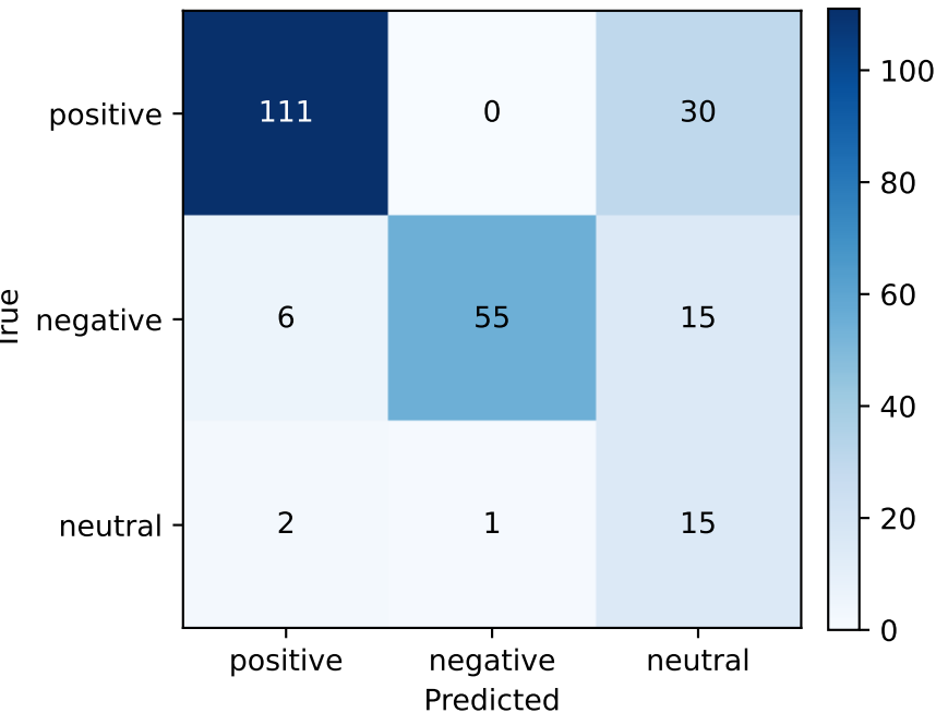
Confusion — FinGPT-Sent (Llama-2-13B)
