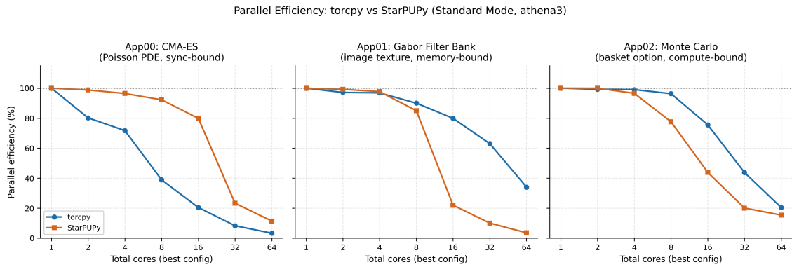
Σχήμα 7.2: Παράμετρος Παραλληλικής Αποδοτικότητας (Parallel Efficiency) για κάθε εφαρμογή και για κάθε αριθμό νήματων εργασίας.
