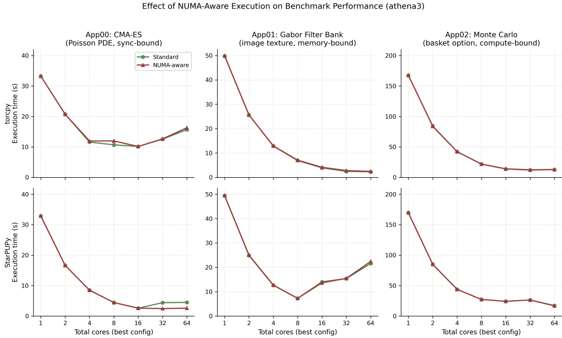
Σχήμα 7.3: Αποτελέσματα Πειραμάτων - NUMA-aware εκτέλεση των εφαρμογών σε σύγκριση με την Standard (NUMA-oblivious) εκτέλεση.
