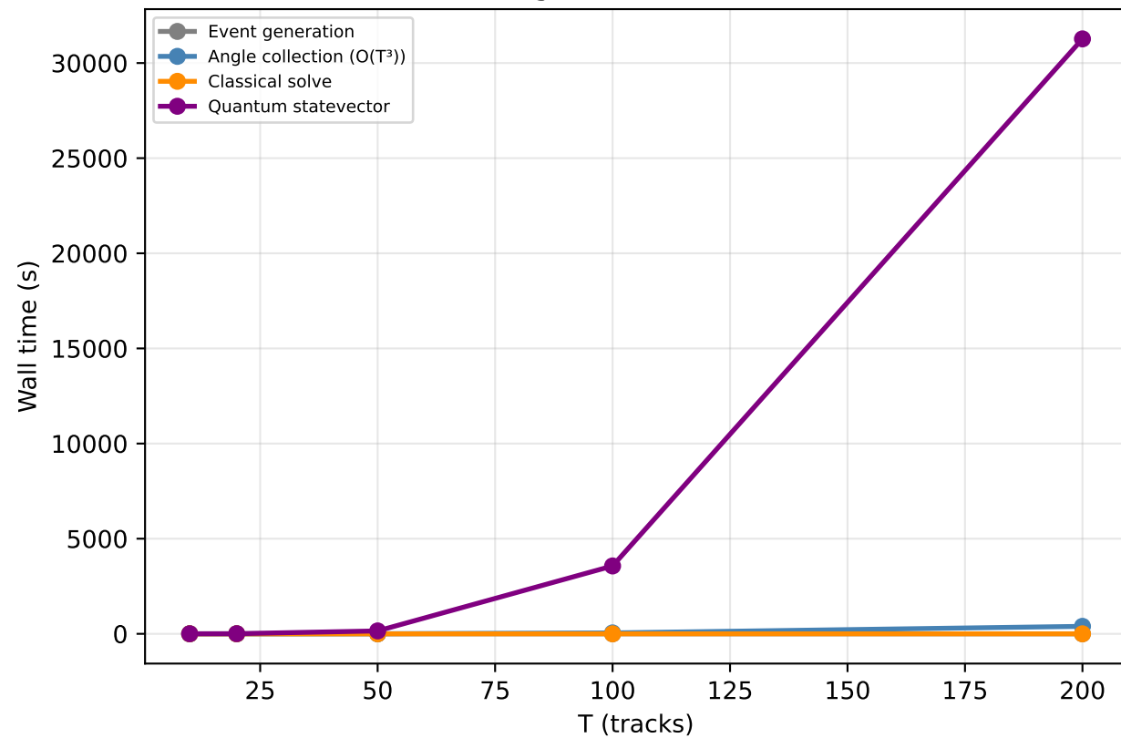
Timing vs T (linear scale)
