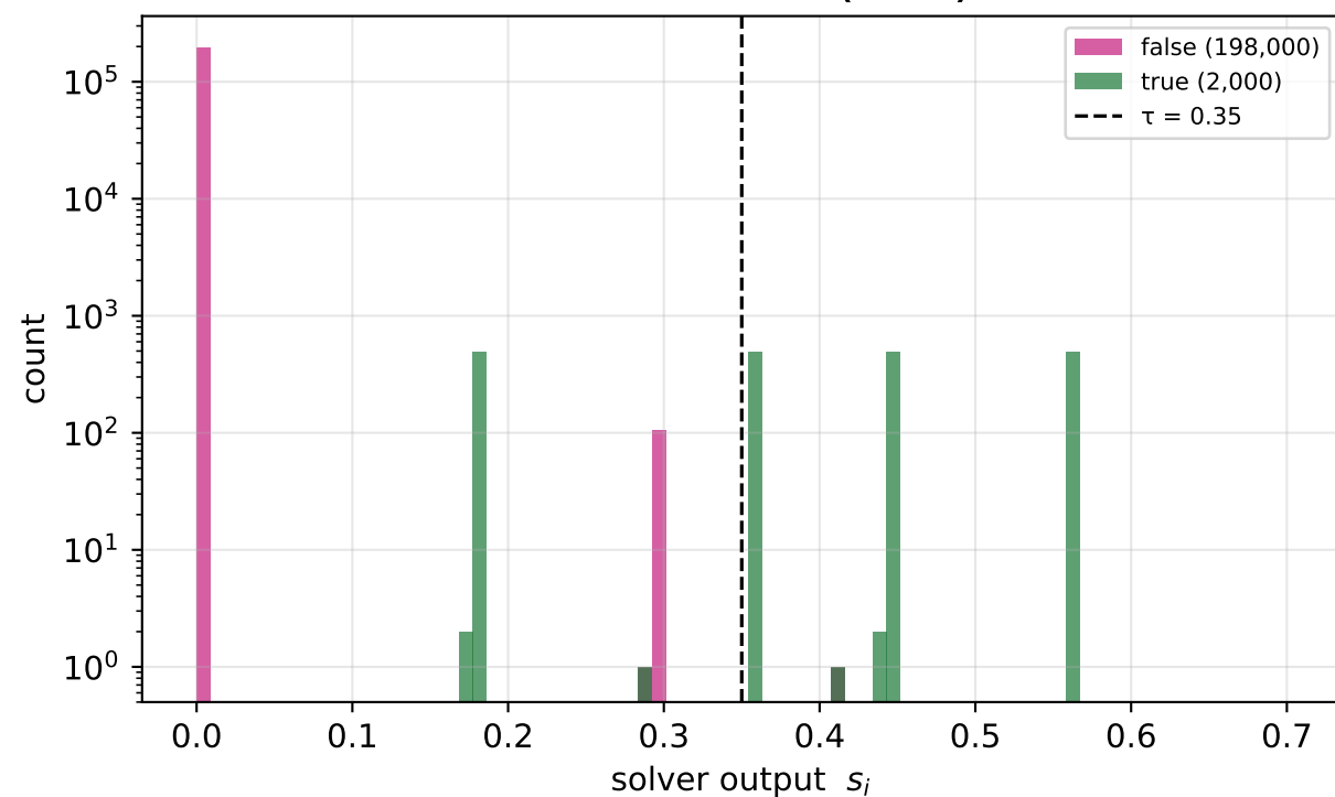
n=100 false> \tau : 1 (0.00%)
