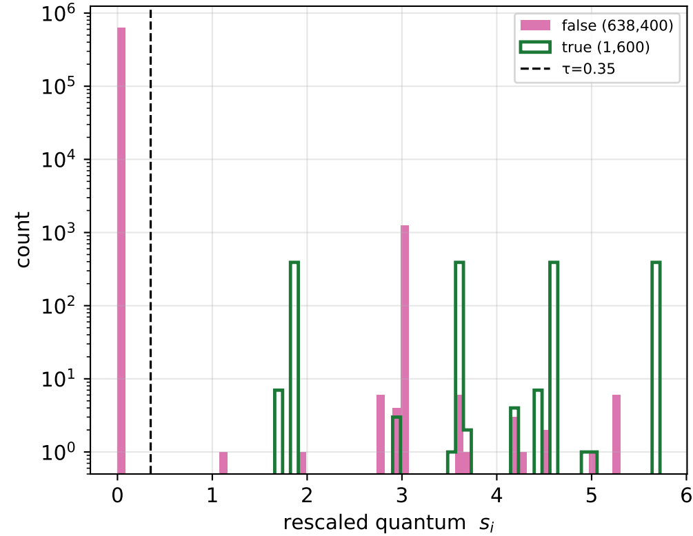
(n=400) false> \tau : 1,289
