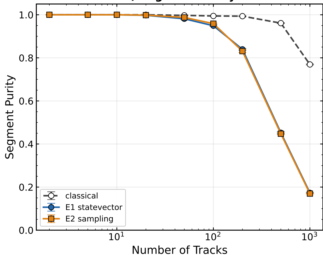
ii) Segment Purity
