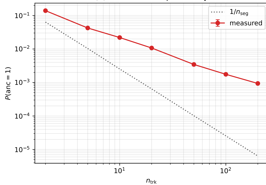
(d) Post-selection probability
