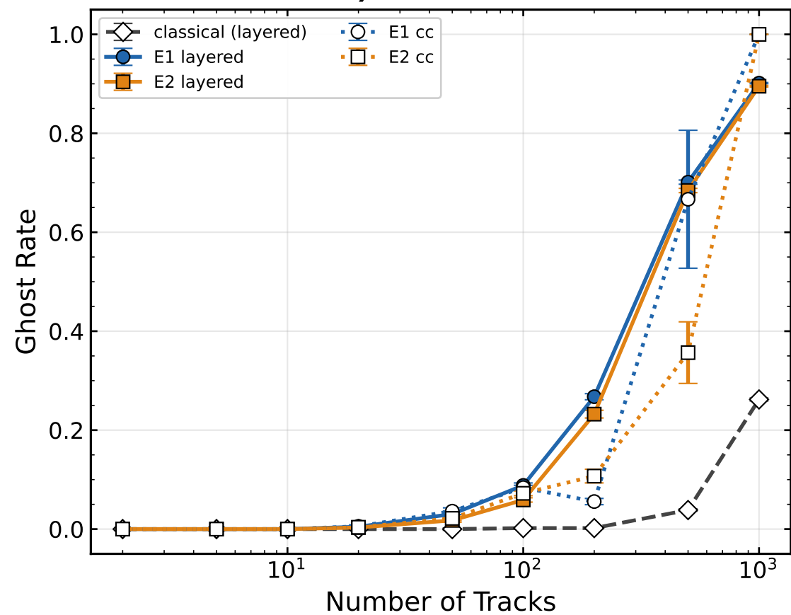
ii) Ghost Rate
