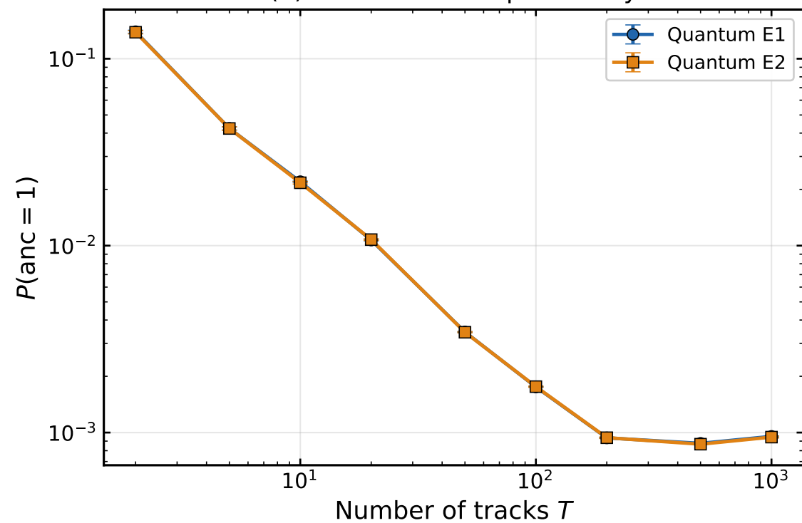
(d) Ancilla success probability
