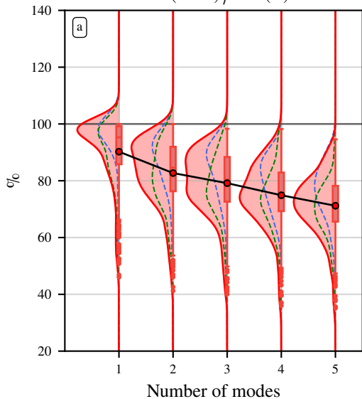
Var(\mathbf{E}^{(m)}) / Var(\mathbf{Y})
