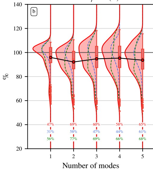
MSE^{(m)} / Var(\mathbf{Y})
