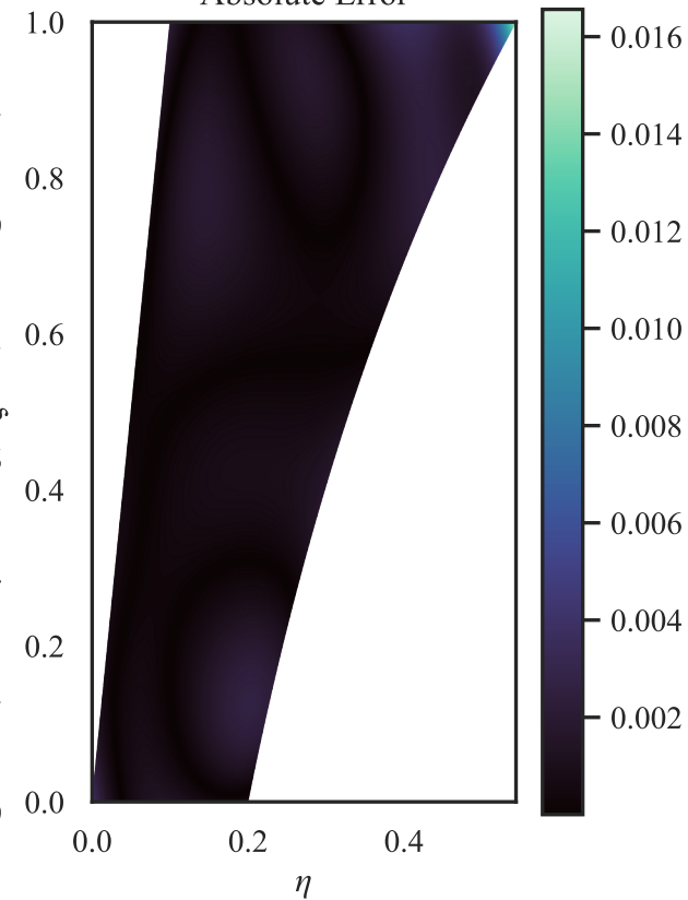
Absolute Error
