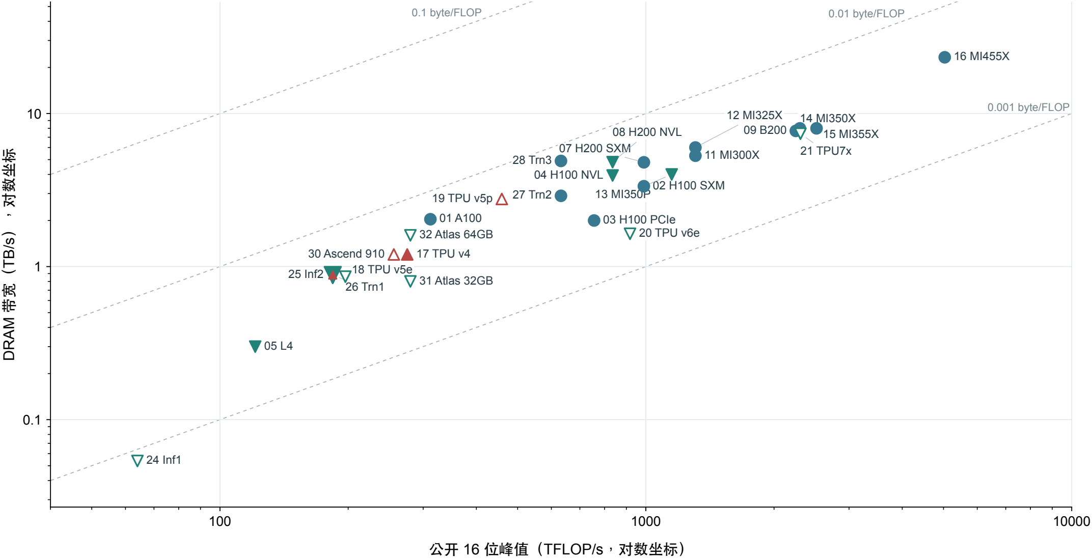
16 位计算峰值与DRAM 带宽：27 个可配对产品
