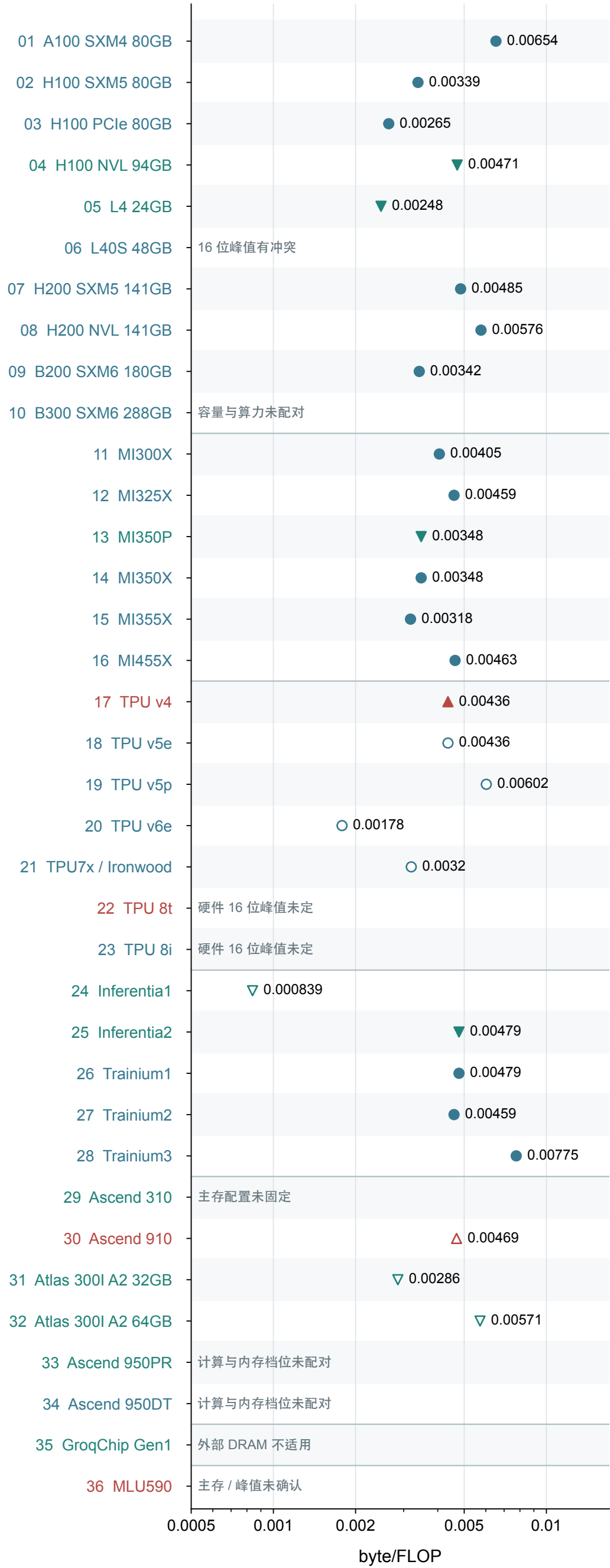
DRAM 带宽 / 16 位峰值
