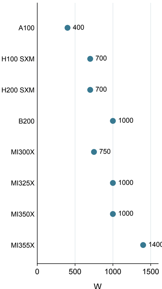
模组上限
