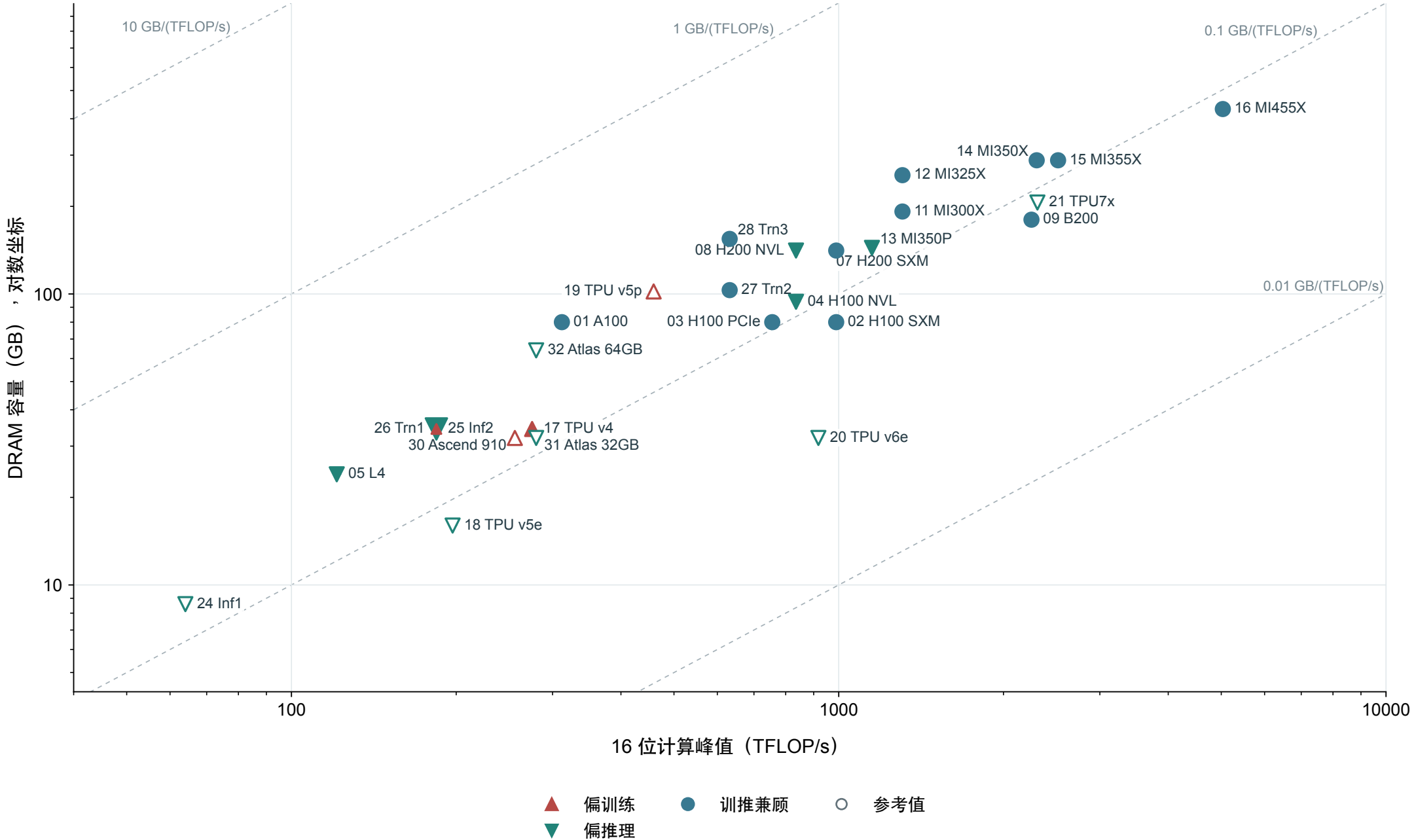
16 位计算峰值与DRAM 容量
