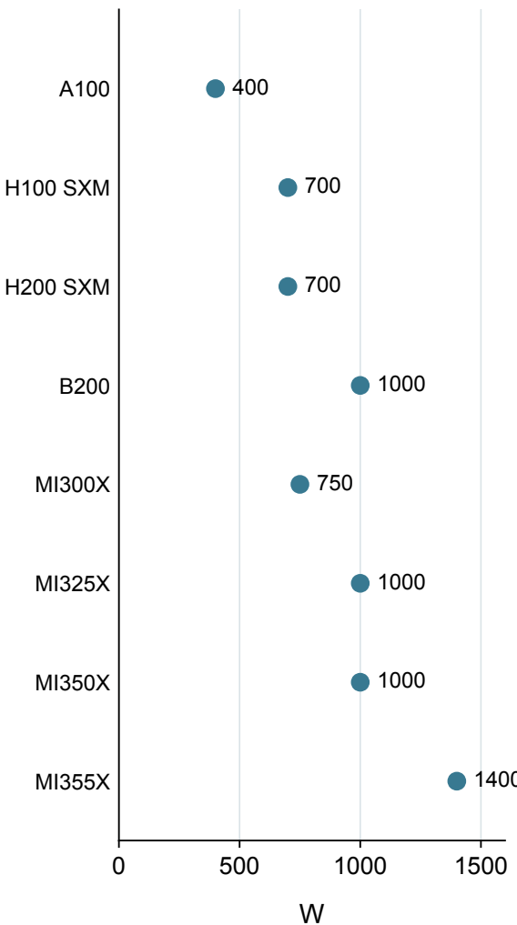
模组上限
