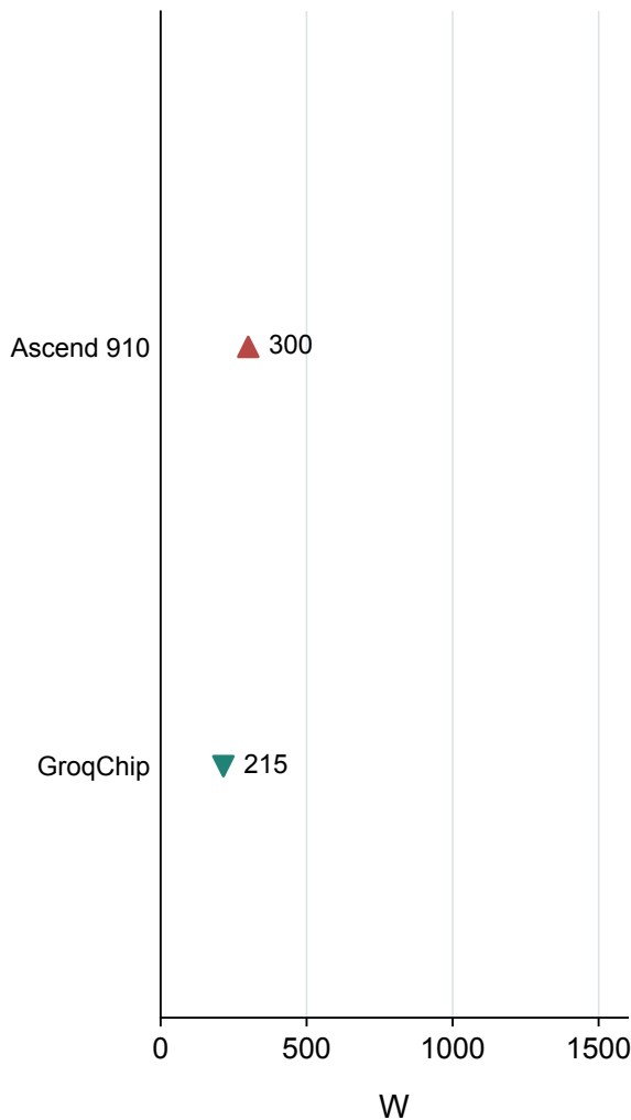
芯片 TDP
