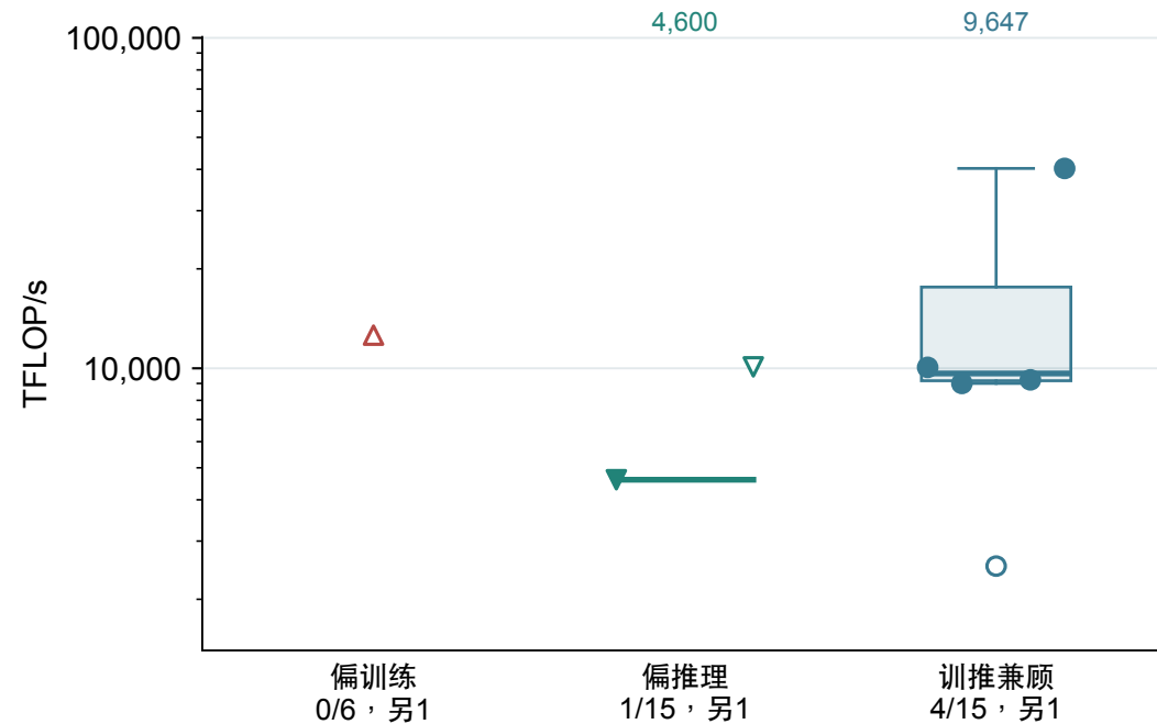
FP4 / MXFP4 矩阵峰值
