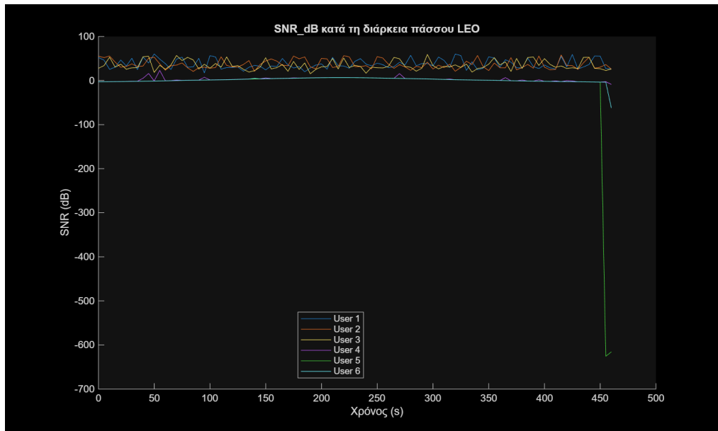
Σχήμα 5.5: SNR του νικητή κόμβου ανά χρήστη κατά τη διάρκεια του πιάσμου. Η απότομη πτώση στο τέλος (χρήστες 5, 6) αντιστοιχεί στο φαινόμενο outage που περιγράφεται στο κείμενο.
