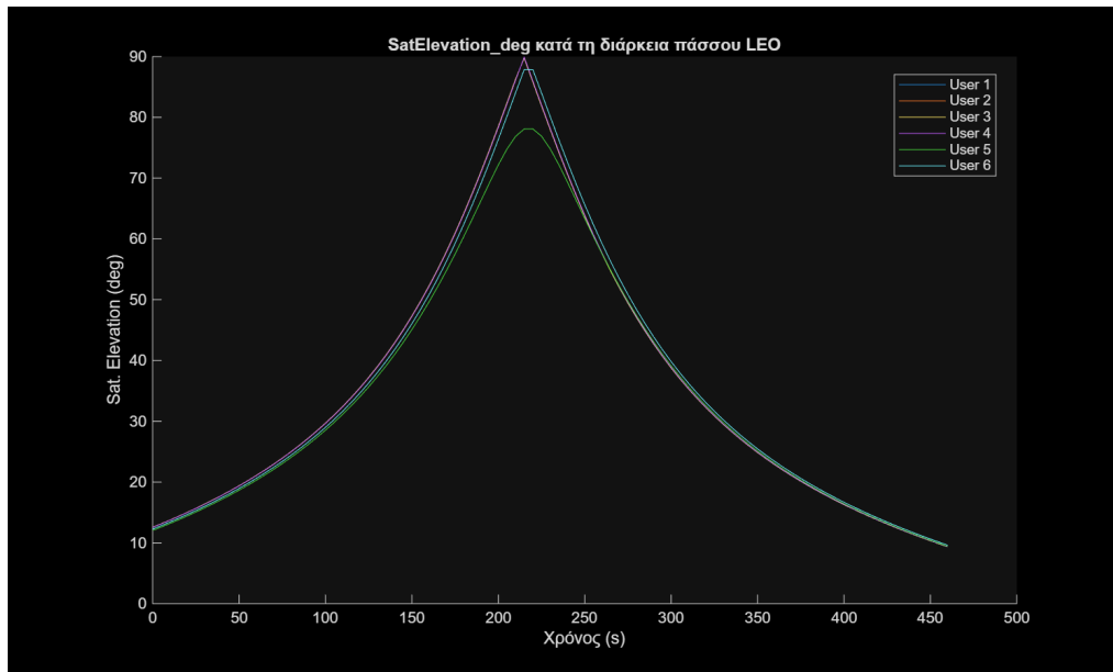
Σχήμα 5.4: Γωνία ανύψωσης δορυφόρου ανά χρήστη κατά τη διάρκεια του πιάσμου (93 βήματα, \Delta t = 5 s).
