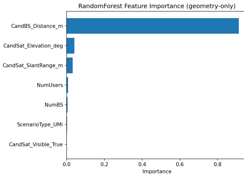
Σχήμα 5.9: Σπουδαιότητα χαρακτηριστικών (Random Forest, μόνο γεωμετρία -- χωρίς SNR ή path loss). Η απόσταση προς το καλύτερο BS κυριαρχεί, αφού είναι πλέον το χαρακτηριστικό που καθορίζει σχεδόν αποκλειστικά αν ένας χρήστης είναι Satellite-only ή DualConnectivity -- βλ. συζήτηση παρακάτω.
