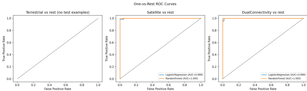
Σχήμα 5.7: One-vs-rest καμπύλες ROC για τα δύο μοντέλα, ανά κλάση. Το υποπλαίσιο Terrestrial δεν έχει καμπύλες, αφού η κλάση αυτή δεν εμφανίζεται στο test set.
