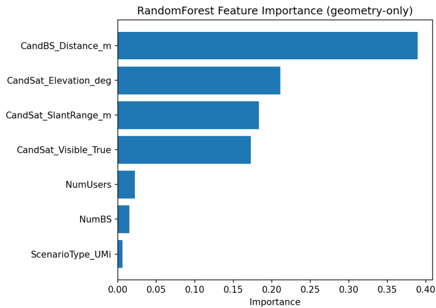
Σχήμα 5.12: Σπουδαιότητα χαρακτηριστικών (Random Forest, μόνο γεωμετρία -- χωρίς SNR ή path loss). Η απόσταση προς το καλύτερο BS παραμένει το πιο σημαντικό χαρακτηριστικό (0.39), αλλά όχι πια συντριπτικά κυρίαρχο: η γωνία ανύψωσης, η slant range και η ορατότητα του δορυφόρου συνεισφέρουν όλες συγκρίσιμα (0.17-0.21 η καθεμία) -- βλ. συζήτηση παρακάτω.
