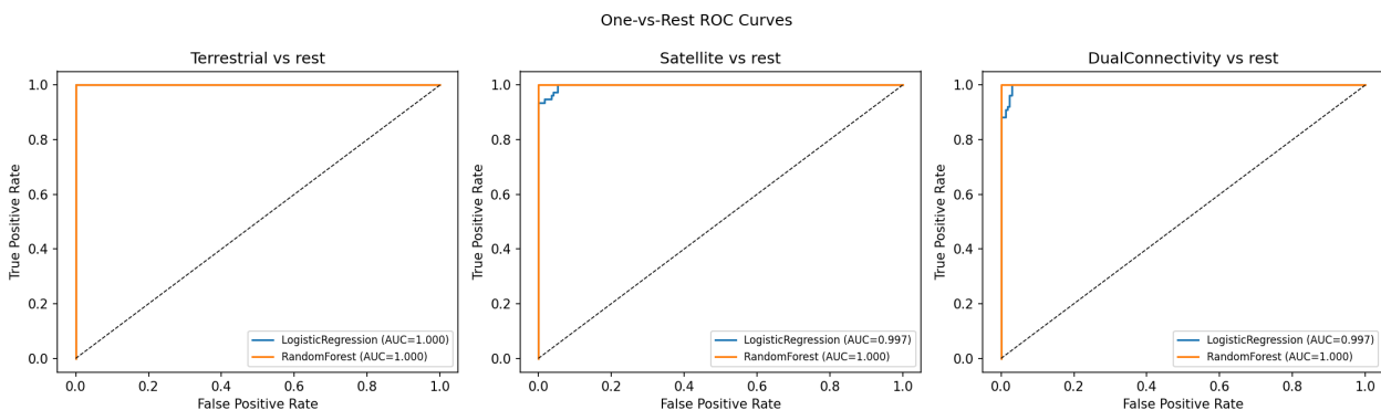
Σχήμα 5.10: One-vs-rest καμπύλες ROC για τα δύο μοντέλα, ανά κλάση. Και οι τρεις κλάσεις έχουν πλέον καμπύλες (η Terrestrial δεν εμφανιζόταν καν στο test set σε παλαιότερη έκδοση αυτού του σχήματος).
