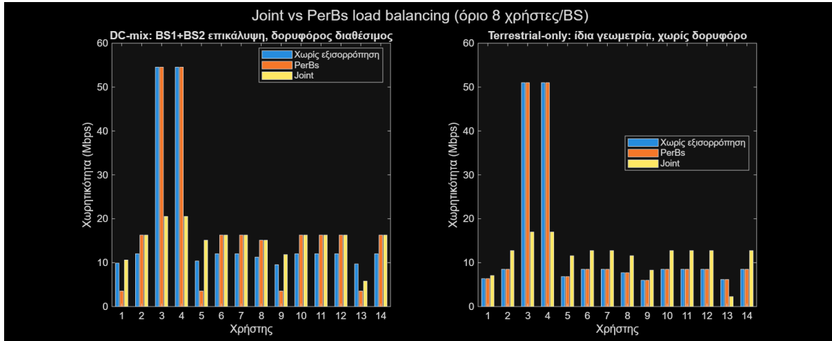
Σχήμα 5.9: Χωρητικότητα ανά χρήστη, jointFairnessDemo.m . Αριστερά: σενάριο DC-mix (δορυφόρος διαθέσιμος παντού). Δεξιά: ίδια γεωμετρία χωρίς δορυφόρο (Terrestrial-only). Σε αμφότερα, "Joint" μετακινεί χρήστες προς τον BS2 αντί να τους αποσυνδέει.
