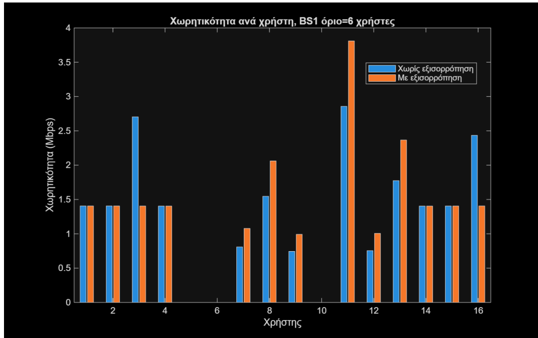
Σχήμα 5.8: Χωρητικότητα ανά χρήστη, χωρίς και με εξισορρόπηση φορτίου ( L_{\max} = 6 ). Οι χρήστες 3 και 16 (DualConnectivity, με δορυφορική εναλλακτική) αποσυνδέονται από τον BS· οι χρήστες 7-9, 11-13 (Terrestrial-only) παραμένουν στον BS με αυξημένο μερίδιο εύρους ζώνης. Οι χρήστες 5, 6, 10 (Outage, καμία εναλλακτική) παραμένουν ανεπηρέαστοι στο μηδέν.
