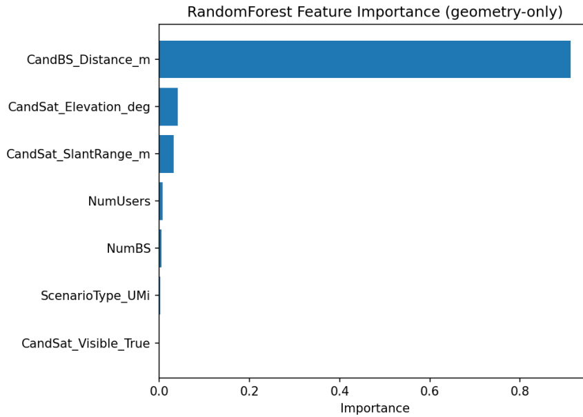
Σχήμα 5.11: Σπουδαιότητα χαρακτηριστικών (Random Forest, μόνο γεωμετρία -- χωρίς SNR ή path loss). Η απόσταση προς το καλύτερο BS κυριαρχεί, αφού είναι πλέον το χαρακτηριστικό που καθορίζει σχεδόν αποκλειστικά αν ένας χρήστης είναι Satellite-only ή DualConnectivity -- βλ. συζήτηση παρακάτω.
