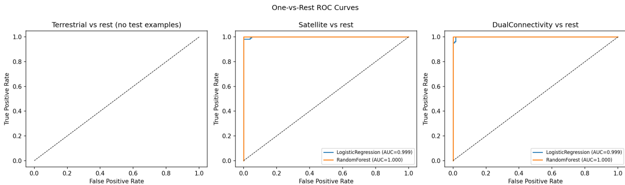
Σχήμα 5.9: One-vs-rest καμπύλες ROC για τα δύο μοντέλα, ανά κλάση. Το υποπλαίσιο Terrestrial δεν έχει καμπύλες, αφού η κλάση αυτή δεν εμφανίζεται στο test set.
