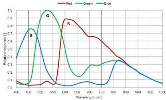
SC230AC/SC230BC量子曲线
