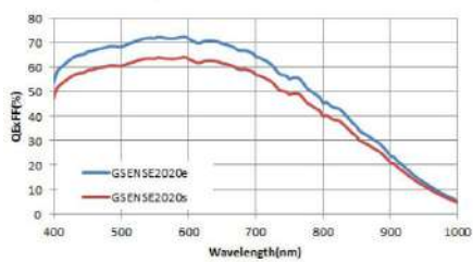
SD400AC/M量子曲线
