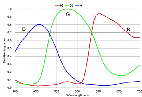
SC2000C量子曲线
