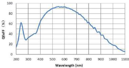
SD400BM量子曲线
