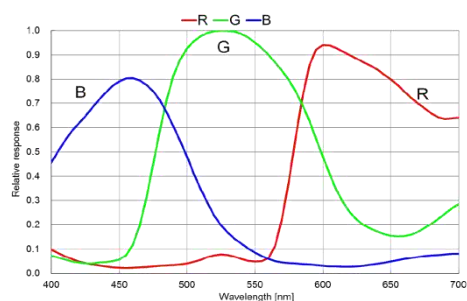
SC600C量子曲线
