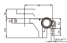
C-FMBN 调焦机构
