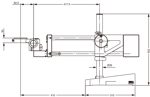
重型万能台架 US-3
