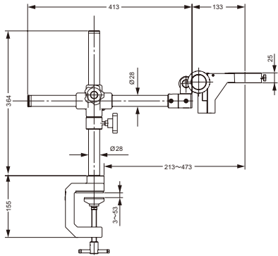
万能台架 G-US2
