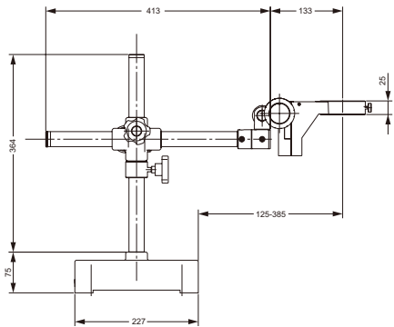
万能台架 G-US2
