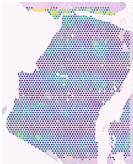
CID4290 | CAFs
