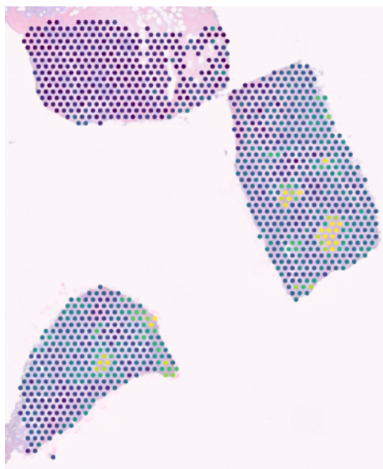
CID44971 | T cells
