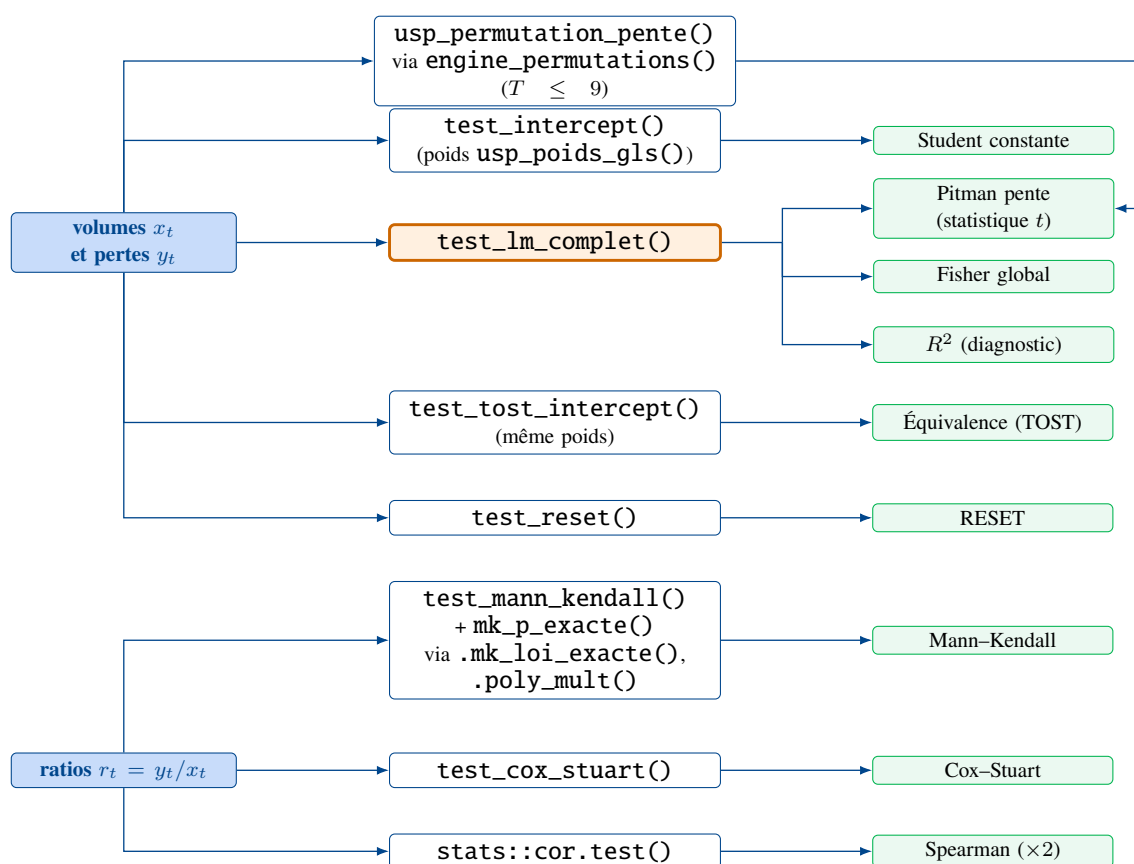
FIGURE 3 : Hypothèse H1. test_lm_complet() alimente deux entrées de la table des tests à partir d'un unique ajustement (Fisher global et R^2 ) et fournit la statistique t de la ligne du test de Pitman sur la pente, dont la p-value vient de usp_permutation_pente() (loi de permutation de Pitman, par énumération des T! appariements à T \leq 9 ou par permutations aléatoires au-delà, issue #169) : une anomalie de cet ajustement fausserait à la fois Fisher, R^2 et la statistique affichée de la pente, une anomalie de usp_permutation_pente() sa p-value. La nullité de la constante utilise les mêmes données, mais tire sa statistique t , ses p-values et, depuis l'issue #215, l'estimation \hat{a}_w affichée sur sa ligne de son propre ajustement, la régression pondérée de test_intercept() (poids d' usp_poids_gls() ); jusqu'à cette issue, l'estimation était lue dans l'ajustement de test_lm_complet() . Le TOST repose sur la même régression pondérée. Les fonctions de régression (constante, test_lm_complet() , TOST, RESET) lisent les volumes et les pertes ( x_t, y_t ); Mann-Kendall, Cox-Stuart et Spearman lisent les ratios r_t , Spearman contre le volume lisant aussi x_t . Mann-Kendall illustre la configuration inverse : un seul test, mais quatre fonctions dont deux internes.
