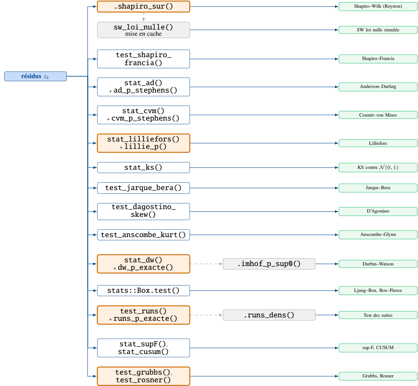
FIGURE 5 : Hypothèses H3 et H4 et diagnostics de stabilité. Tous les tests partent du même objet, les résidus z_t : une erreur dans usp_noyau() affecterait l'intégralité de ce graphe. Trois fonctions internes (en gris) fournissent des lois de référence : sw_loi_nulle() , .imhof_p_sup0() et .runs_dens() . .shapiro_sur() alimente deux entrées distinctes de la table des tests.
