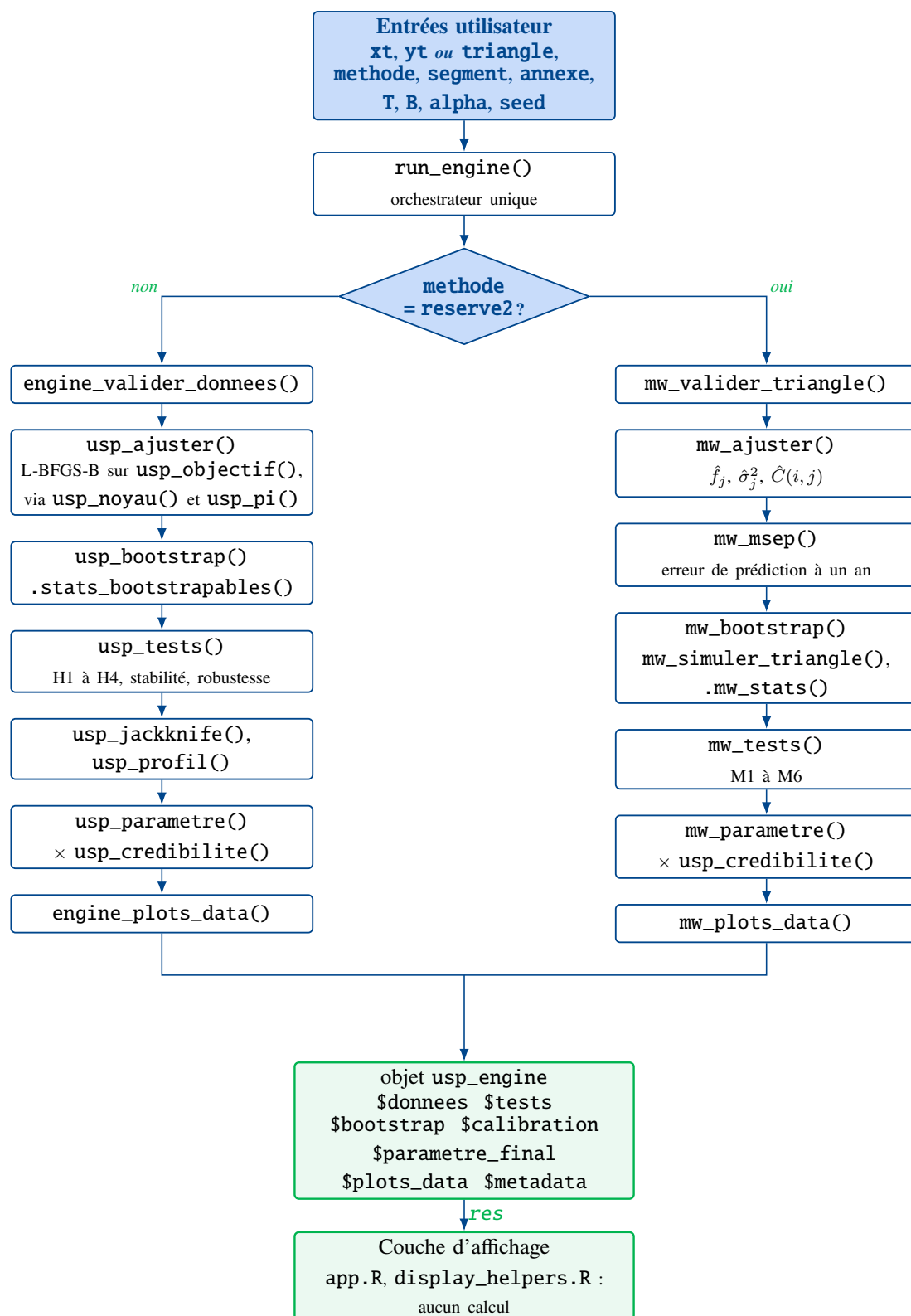
FIGURE 1 : Architecture du moteur R/engine.R. Le paramètre methode aiguille vers l’une des deux chaînes : à gauche les méthodes lognormales (sections B et C de l’annexe XVII), à droite la méthode Merz–Wüthrich (section D). Les deux convergent vers un objet de sortie unique, que la couche d’affichage se contente de lire. usp_credibilite() est la seule fonction de calcul partagée par les deux branches.
