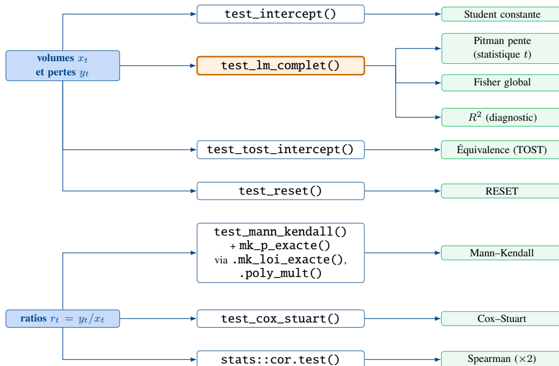
FIGURE 3 : Hypothèse H1. test_lm_complet() alimente deux entrées de la table des tests à partir d'un unique ajustement (Fisher global et R^2 ) et fournit la statistique t de la ligne du test de Pitman sur la pente, dont la p-value vient de usp_permutation_pente() : une anomalie de cet ajustement fausserait à la fois Fisher, R^2 et la pente. La nullité de la constante utilise les mêmes données, mais tire sa statistique t et ses p-values de son propre ajustement, test_intercept() ; seule l'estimation \hat{a} affichée sur sa ligne est lue dans l'ajustement de test_lm_complet() . Les fonctions de régression (constante, test_lm_complet() , TOST, RESET) lisent les volumes et les pertes ( x_t, y_t ) ; Mann-Kendall, Cox-Stuart et Spearman lisent les ratios r_t , Spearman contre le volume lisant aussi x_t . Mann-Kendall illustre la configuration inverse : un seul test, mais quatre fonctions dont deux internes.
