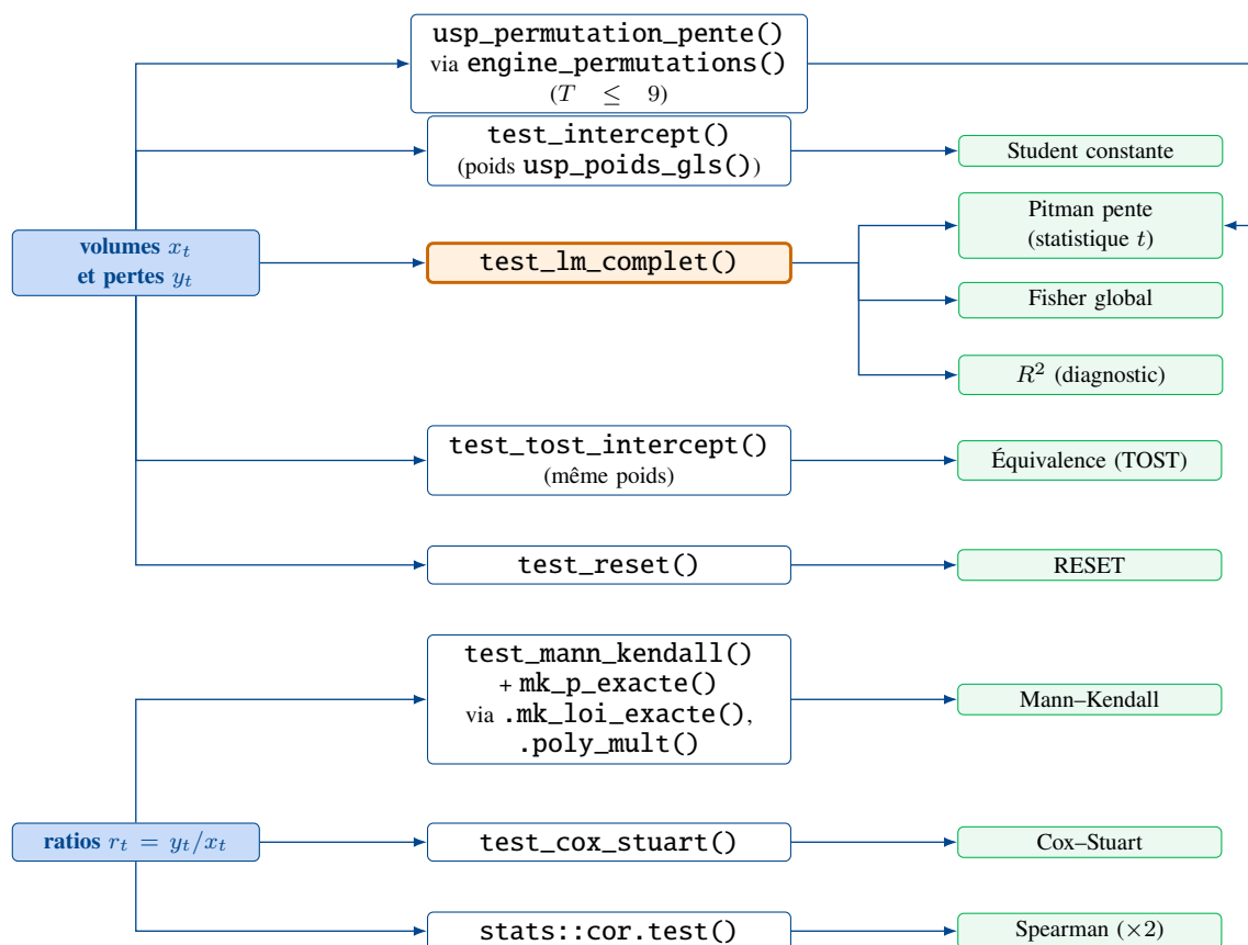
FIGURE 3 : Hypothèse H1. test_lm_complet() alimente deux entrées de la table des tests à partir d'un unique ajustement (Fisher global et R^2 ) et fournit la statistique t de la ligne du test de Pitman sur la pente, dont la p-value vient de usp_permutation_pente() (loi de permutation de Pitman, par énumération des T! appariements à T \leq 9 ou par permutations aléatoires au-delà, issue #169) : une anomalie de cet ajustement fausserait à la fois Fisher, R^2 et la statistique affichée de la pente, une anomalie de usp_permutation_pente() sa p-value. La nullité de la constante utilise les mêmes données, mais tire sa statistique t , ses p-values et, depuis l'issue #215, l'estimation \hat{a}_w affichée sur sa ligne de son propre ajustement, la régression pondérée de test_intercept() (poids d' usp_poids_gls() ); jusqu'à cette issue, l'estimation était lue dans l'ajustement de test_lm_complet() . Le TOST repose sur la même régression pondérée. Les fonctions de régression (constante, test_lm_complet() , TOST, RESET) lisent les volumes et les pertes ( x_t, y_t ); Mann-Kendall, Cox-Stuart et Spearman lisent les ratios r_t , Spearman contre le volume lisant aussi x_t . Mann-Kendall illustre la configuration inverse : un seul test, mais quatre fonctions dont deux internes.
