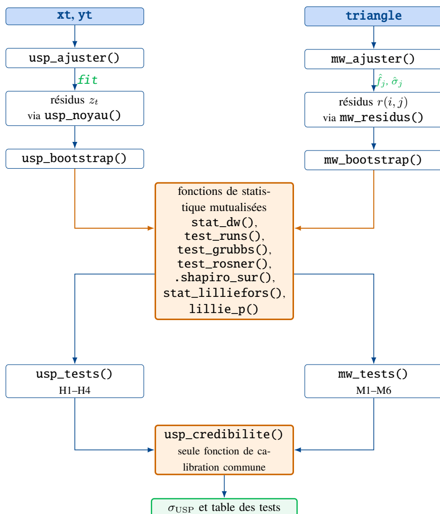
FIGURE 2 : Vue chapeau. Les deux branches sont disjointes jusqu'aux fonctions de statistique, dont sept sont mutualisées (en orange), puis se rejoignent sur usp_credibilite(). Une anomalie dans un bloc orange affecterait les deux méthodes.
