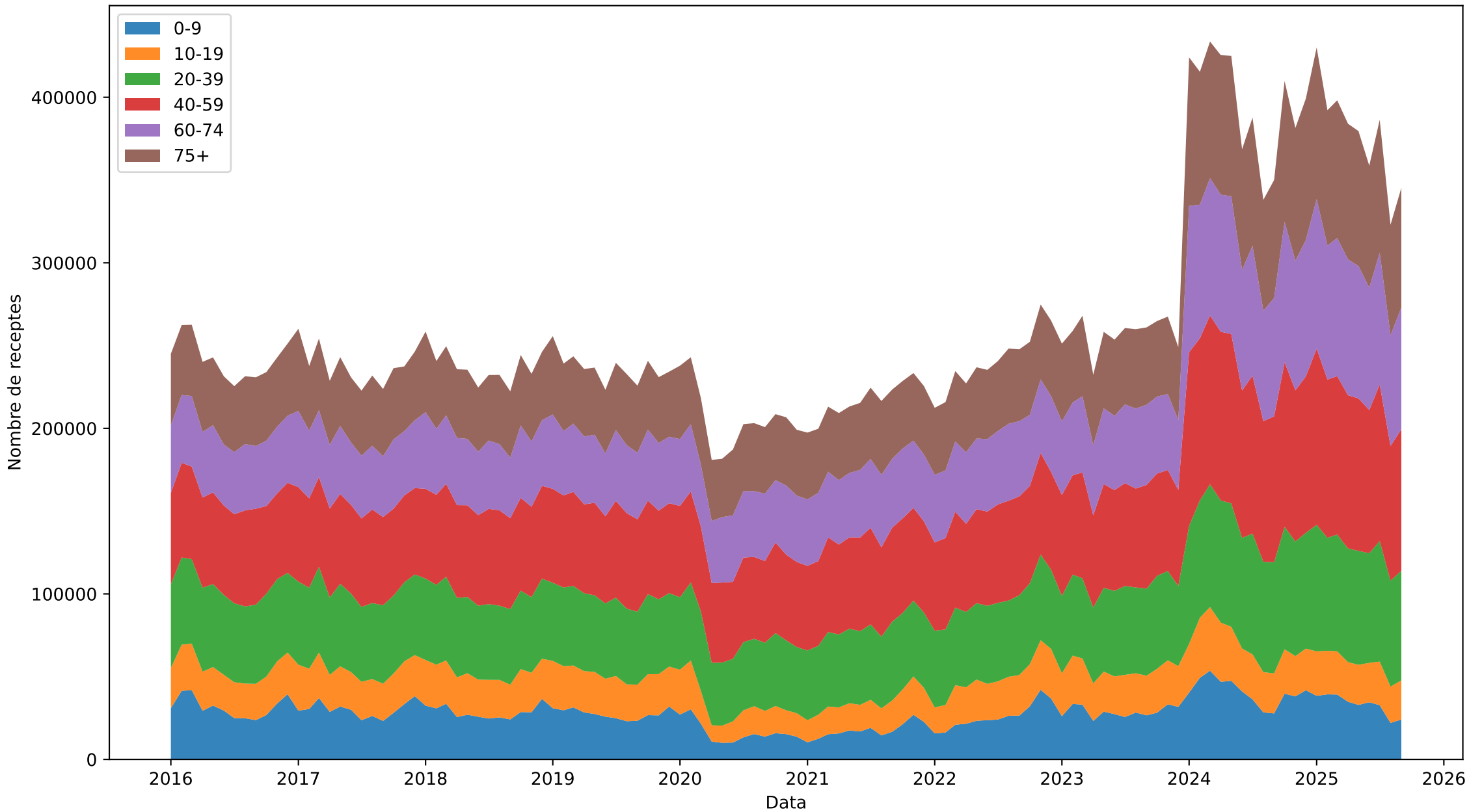
Evolució temporal de receptes per grup d'edat — ATC1 = ANTIINFECCIOSOS PARA USO SISTEMICO
