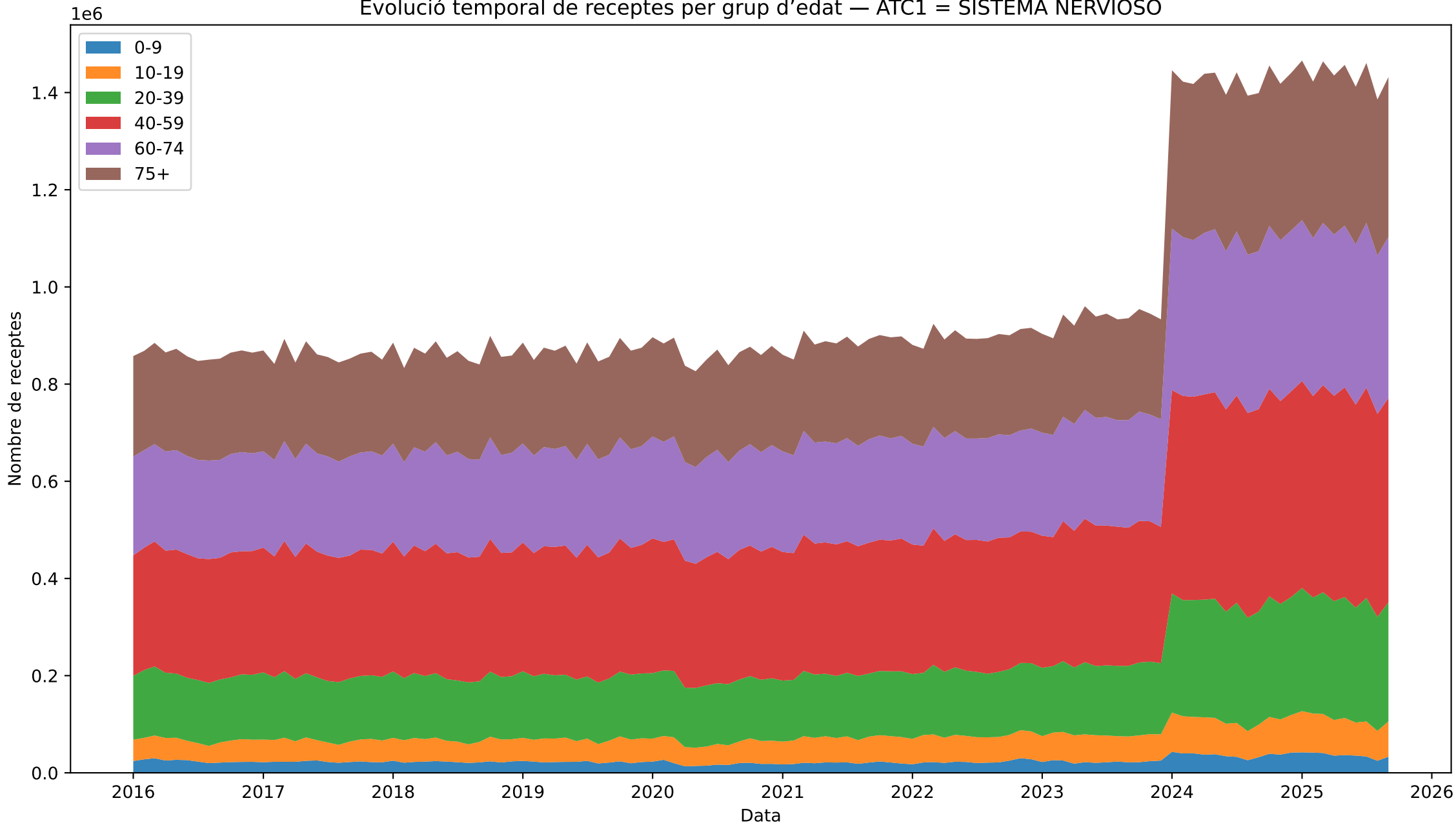
Evolució temporal de receptes per grup d'edat — ATC1 = SISTEMA NERVIOSO
