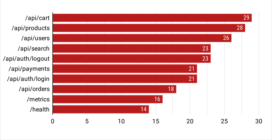
Errores 5xx según endpoint
