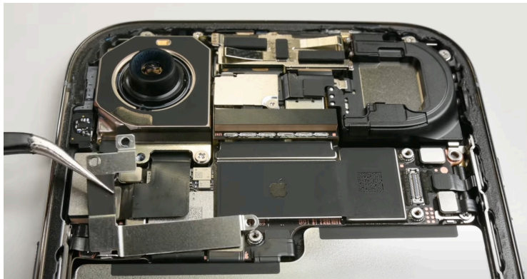
Figura X. Distribución interna de los componentes del iPhone Air. Imagen de iFixit, reproducida en iPhoneros (2025).
