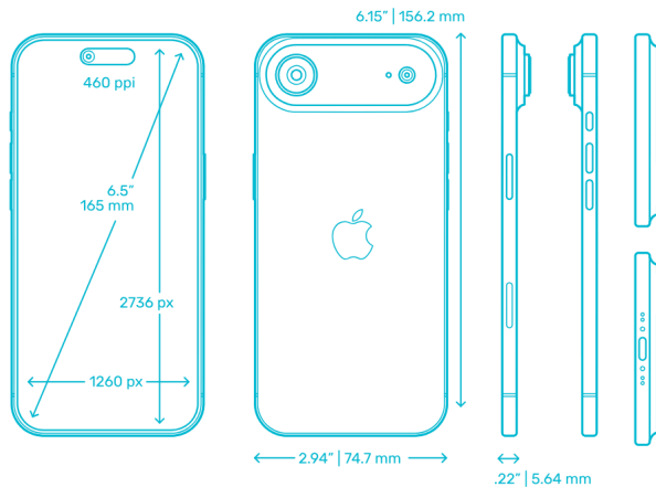
Figura 1. Dimensiones físicas del iPhone Air.
