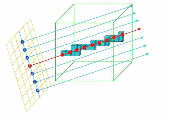
Figura 1.2: Proceso de Raymarching
