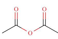
acetic-anhydride
