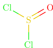
thionyl-chloride
