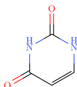
uracil
