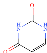
uracil
