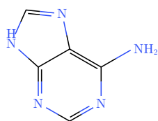
uracil
