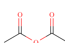
acetic-anhydride
