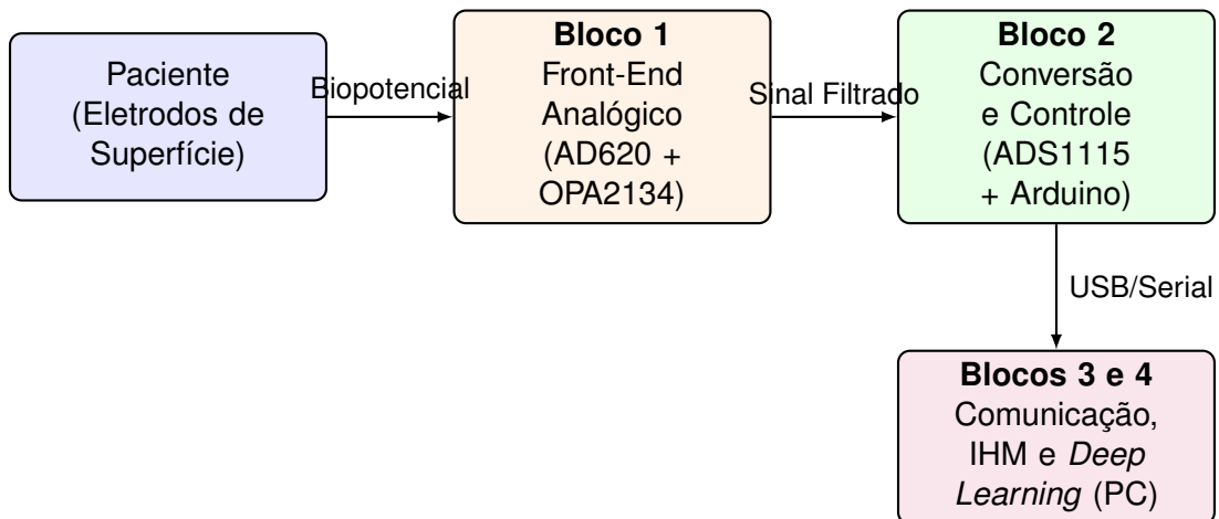
Figura 4 – Diagrama de blocos geral da plataforma híbrida de instrumentação, ilustrando o fluxo do sinal desde a aquisição analógica até o processamento computacional.
