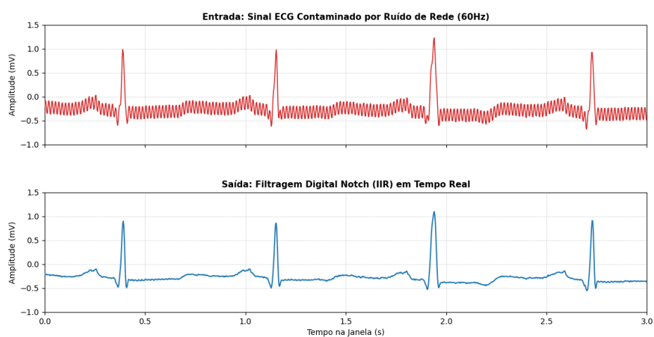
Figura 6 – Comparativo de Filtragem Digital. A) Sinal de entrada contaminado por ruído de rede de 60 Hz. B) Sinal de saída após aplicação do filtro IIR Notch em tempo real, recuperando a morfologia do ECG.
