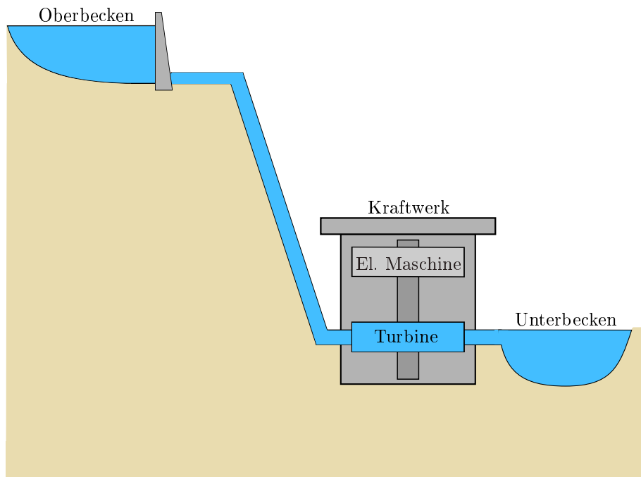
Abbildung 2.1: Pumpspeicherkraftwerk. Aufbau mit Ober- und Unterbecken, Turbinen und elektrischer Maschine zur Energiespeicherung und Rückgewinnung.
