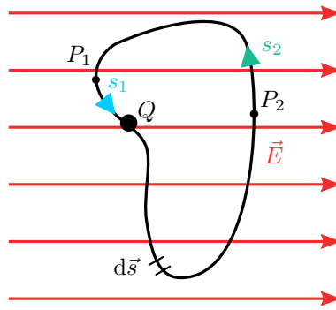
Abbildung 2.6: Bewegung einer Punktladung. Zeigt die Bewegung einer Punktladung entlang zweier Strecken. Die Arbeit die verrichtet wird entlang einer geschlossenen Strecke in einem statischen elektrischen Feld ist Null.
