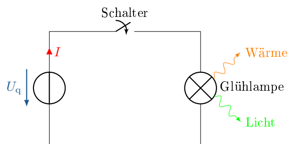
Abbildung 2.8: Beispielschaltung zum Wirkungsgrad. Zeigt die Abgabe von Wärme und Licht am Verbraucher. Das Verhältnis von Licht zu Wärme entspricht dem Wirkungsgrad.
