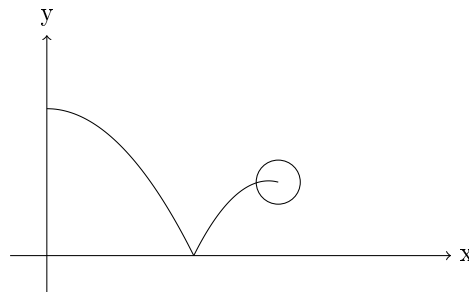
Abbildung 2.2: Energieerhaltungssatz. Die potentielle Energie des Balls wird während des Fallens in kinetische Energie umgewandelt. Beim Aufprall geht ein Teil dieser Energie als Verluste verloren. Der Gesamtenergiegehalt bleibt dennoch konstant.
