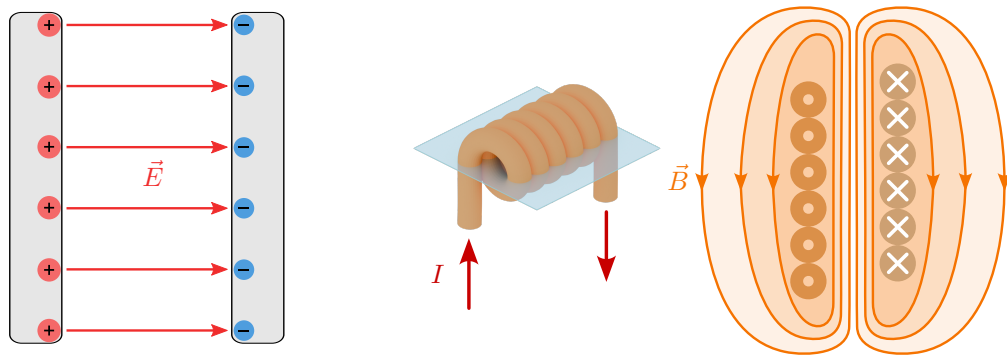
Abbildung 2.4: Elektrische Energiespeicher. Ein idealer Plattenkondensator (links) speichert die Energie im elektrischen Feld, eine ideale Spule (rechts) speichert die Energie im magnetischen Feld.
