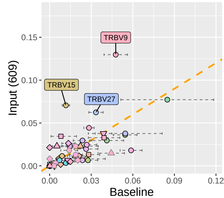
TRBV
