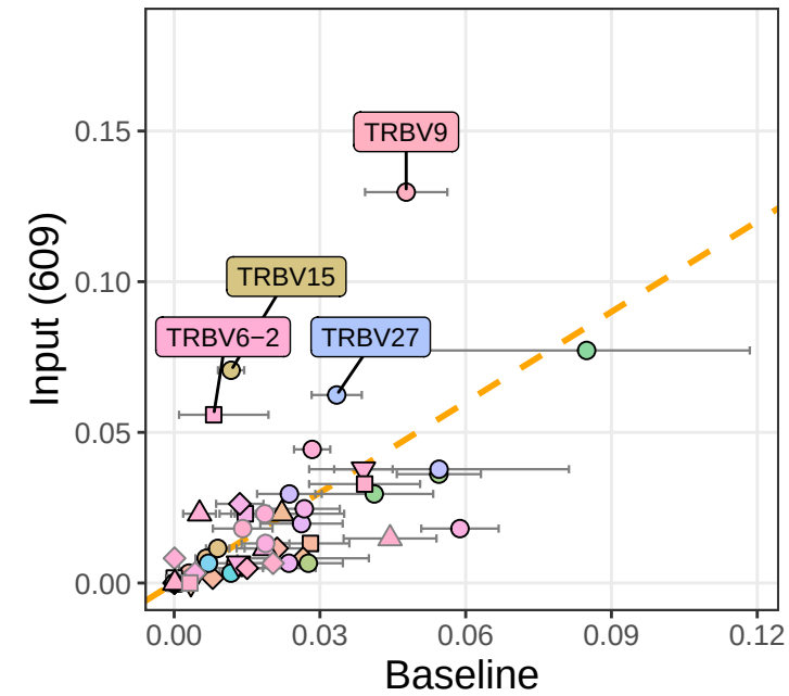
TRBV
