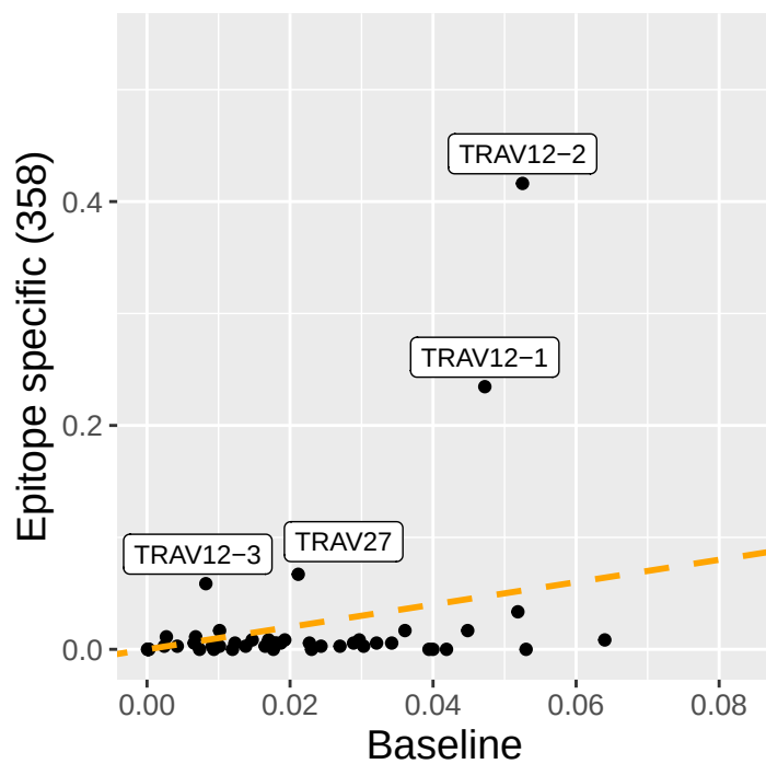
TRAV
