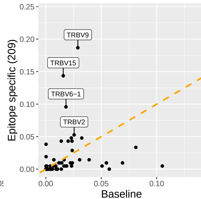
TRBV
