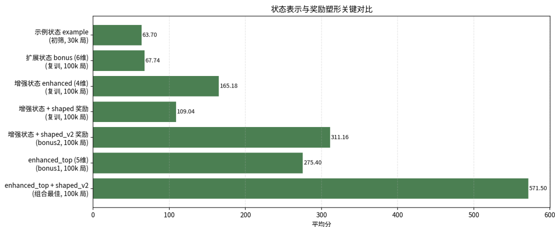
图 5: 状态表示与奖励塑形关键对比
