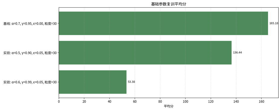
图 2: 基础参数复训结果
