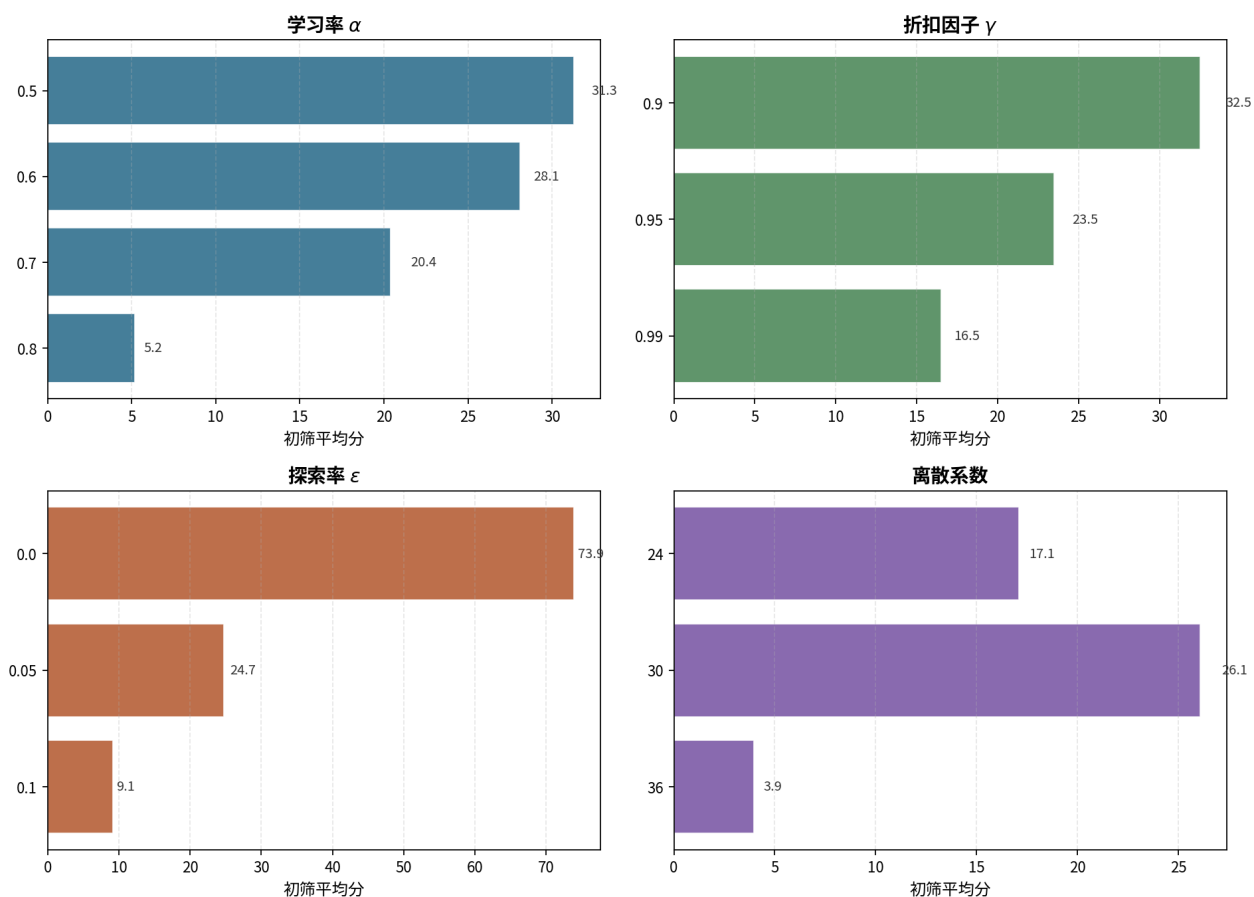
图 4: 各参数对初筛性能的影响（基于 18 组 30k 局训练，按参数值分组取平均）
