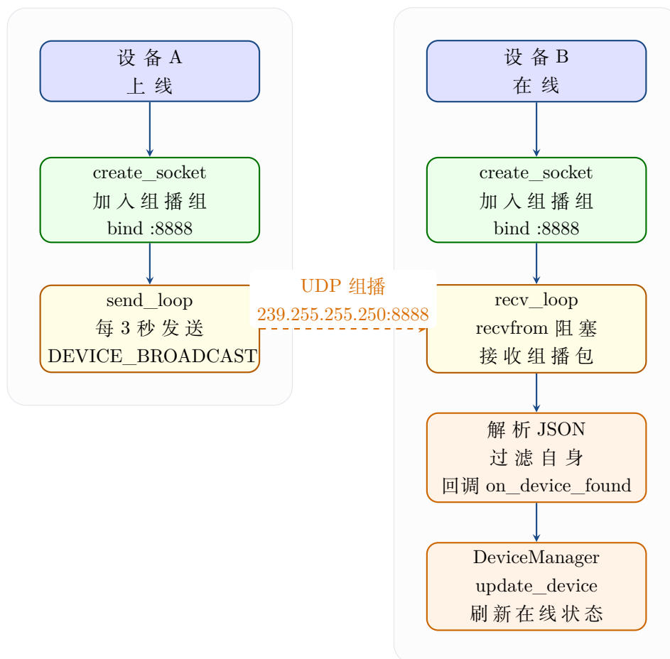
图 2: UDP 组播设备发现流程
