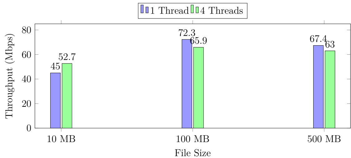
图 7: 不同文件大小与线程数的吞吐量对比
