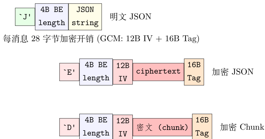
图 4: 数据通道加密线格式
