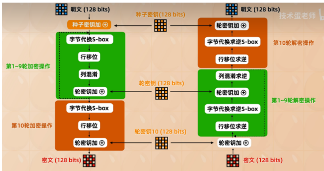
图 3: AES 加密流程
