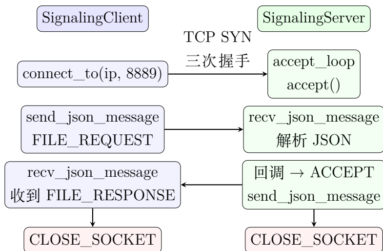
图 5: 信令通道短连接请求-响应流程 (以 FILE_REQUEST 为例)
