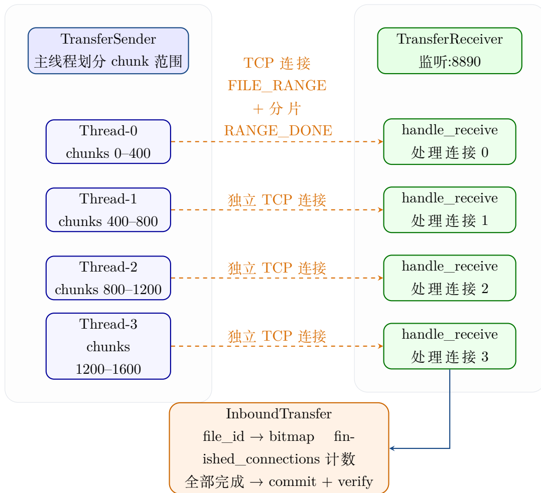
图 6: 多线程并行传输时序图 (4 线程, 1600 chunks, 每个线程 400 chunks)
