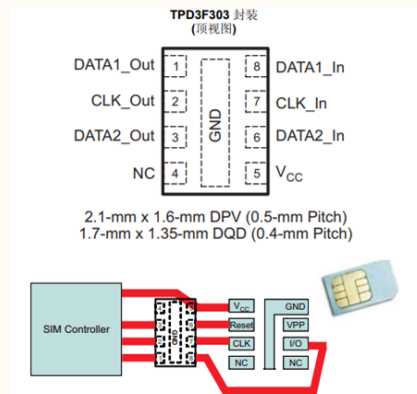
图 1. 在 SIM 卡接口上使用 TPD3F303 的电路板布局
