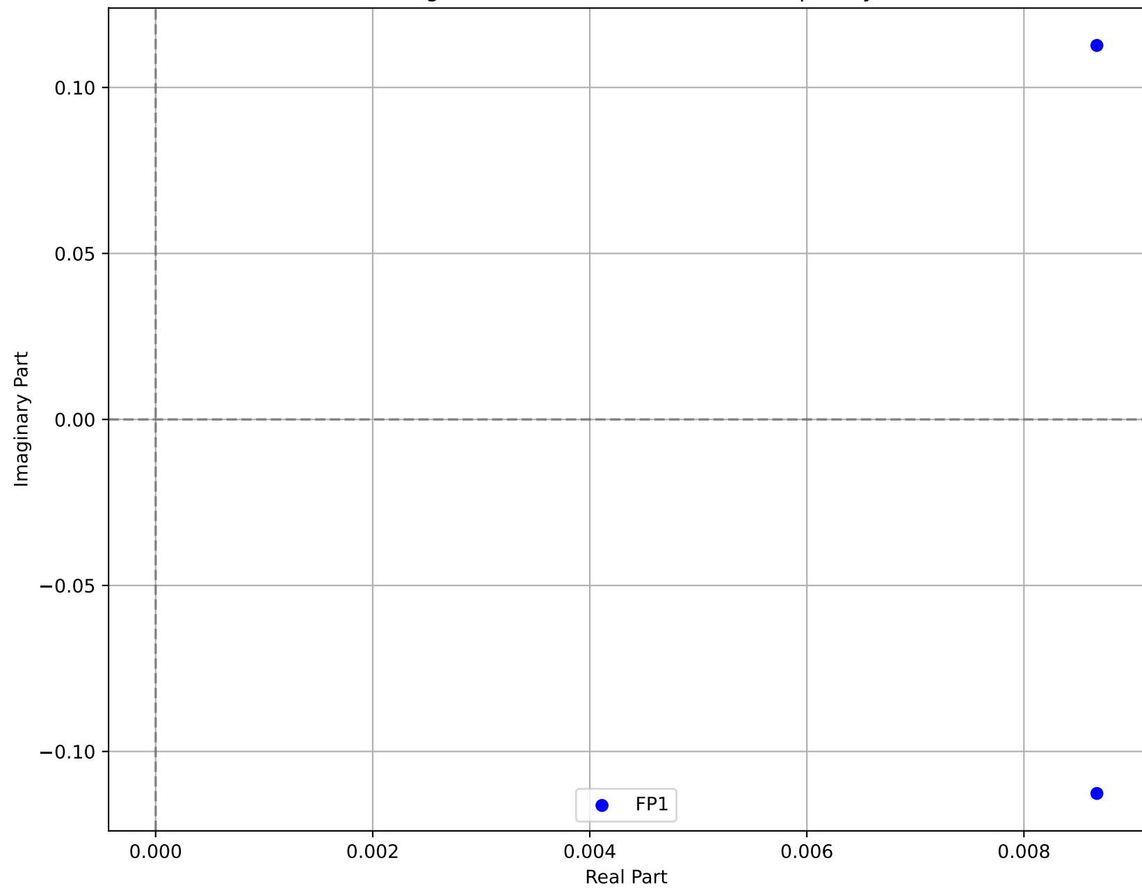
Unstable Eigenvalues for Task 0 ( \omega=0.100 , Sparsity=0.00)
