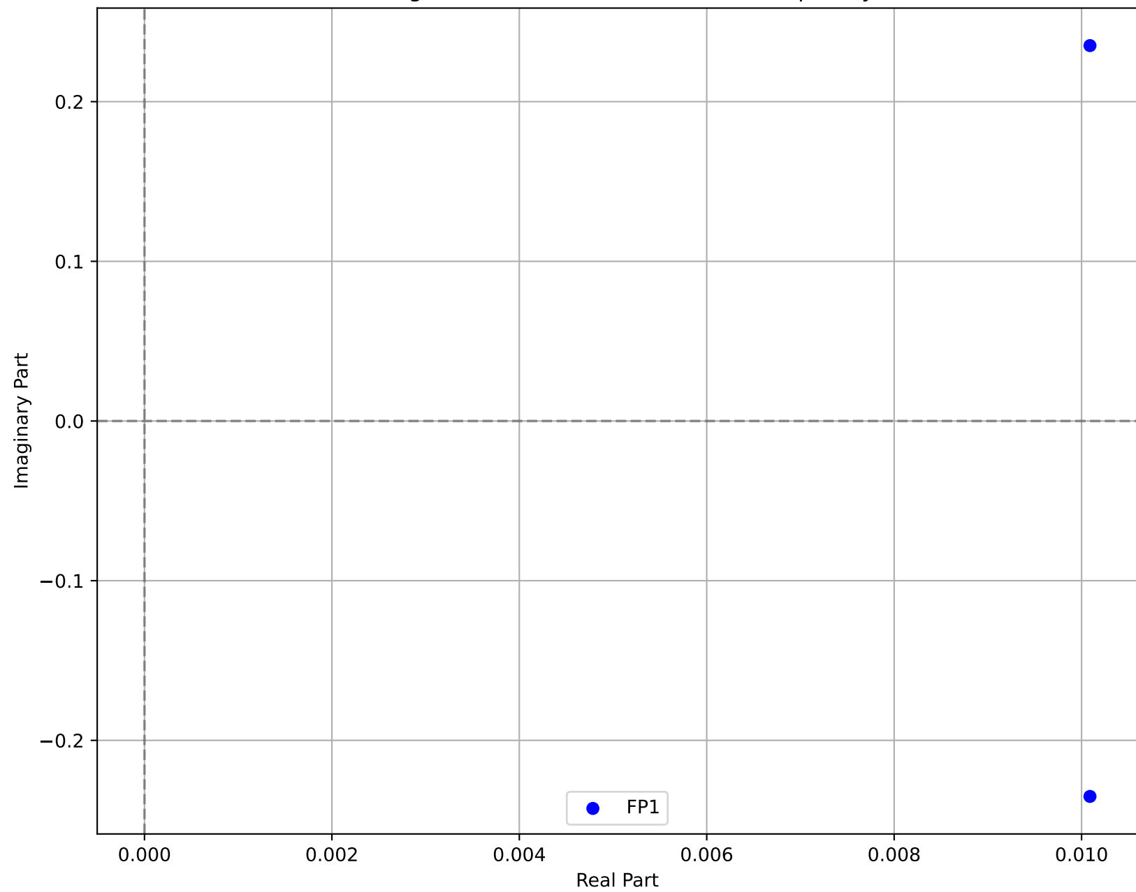
Unstable Eigenvalues for Task 12 ( \omega=0.220 , Sparsity=0.00)
